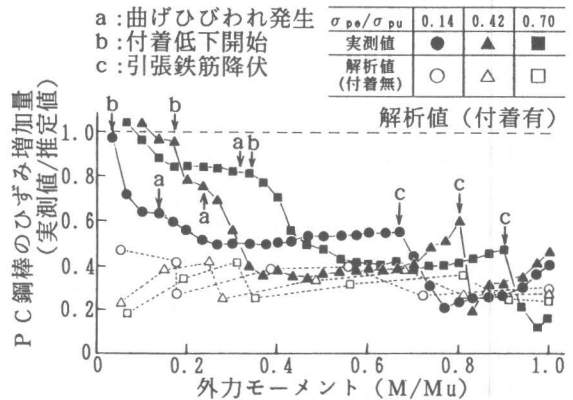
図-8 P C 鋼棒の付着性能 (矩形断面)
