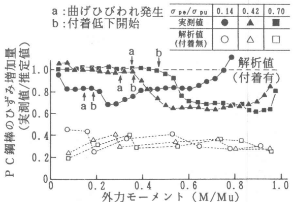
図-9 P C 鋼棒の付着性能 (T形断面)
