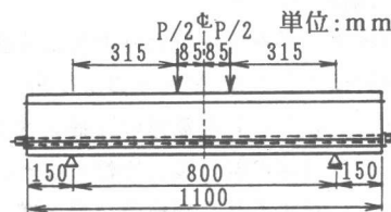
図-2 荷重方法
