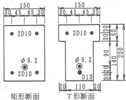
図-1 断面形状 単位:mm
