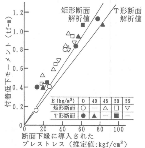
図-11 断面下縁に導入されたプレストレスと付着低下モーメントとの関係
