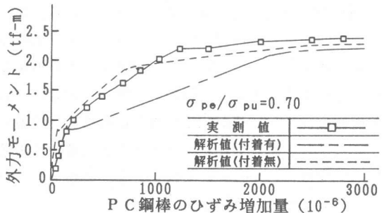
図-5 P C 鋼棒のひずみ変化 (T形断面)
