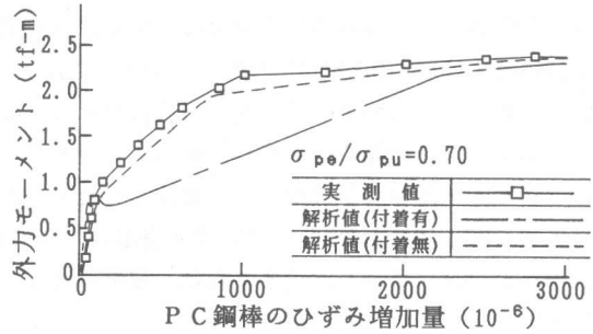
図-4 P C 鋼棒のひずみ変化 (矩形断面)
