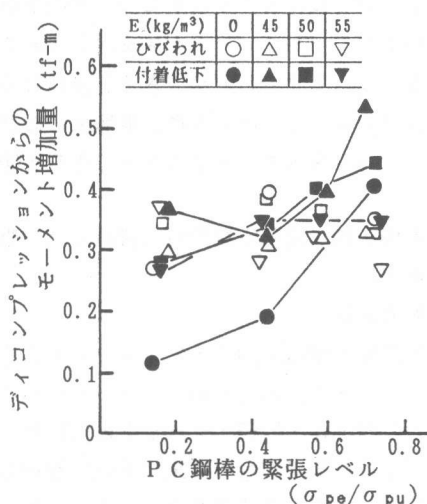
図-10 付着低下モーメント（矩形断面）
