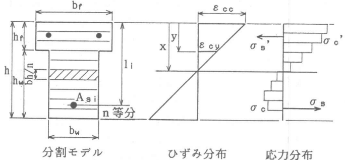
図-3 曲げ解析に用いた積層モデルの説明図
