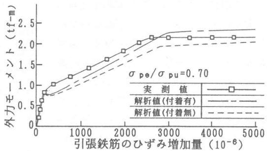
図-6 引張鉄筋のひずみ変化 (矩形断面)
