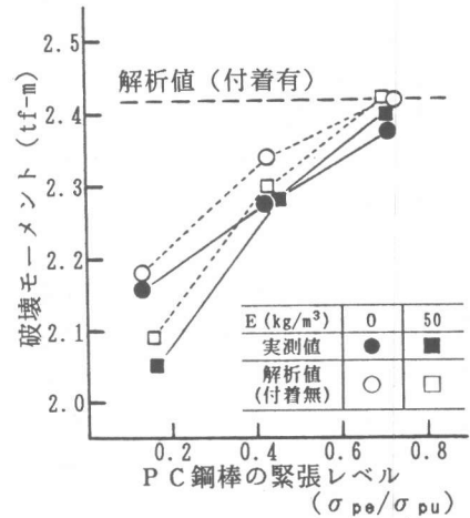
図-7 破壊モーメント (矩形断面)
