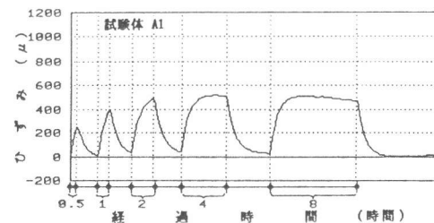
図10 張り付けモルタルの実ひずみ経時変化
