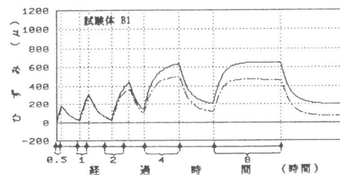
図11 下地モルタルの実ひずみ経時変化
