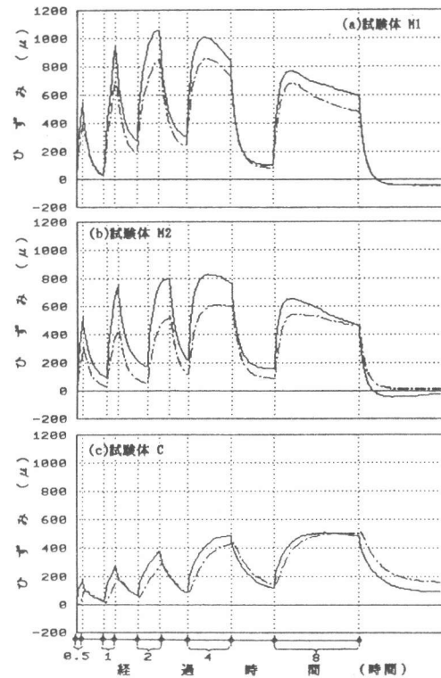
図6 試験体実ひずみの経時変化
