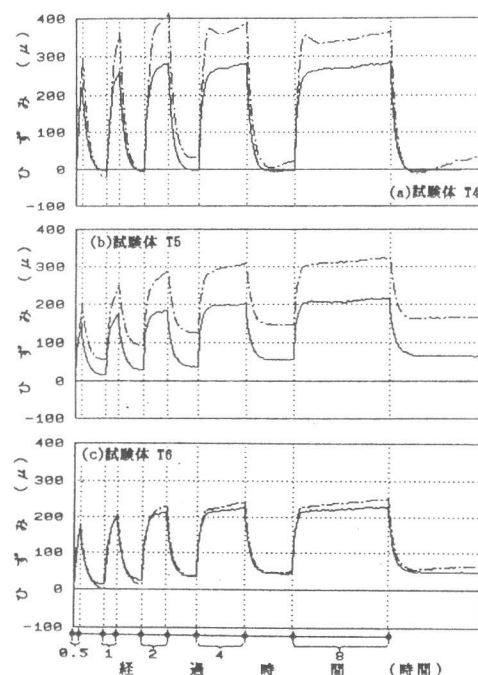
図4 試験体実ひずみの経時変化
