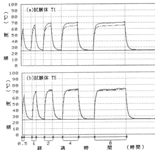
図2 試験体の温度の経時変化
