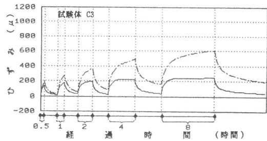
図12 試験体実ひずみの経時変化
