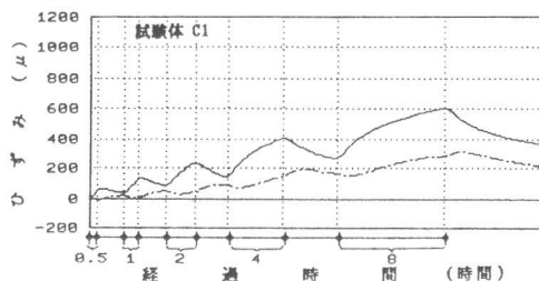
図9 コンクリート部分の実ひずみ経時変化
