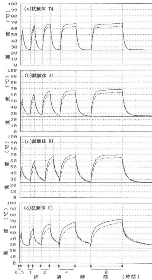
図7 タイル部分の温度経時変化
