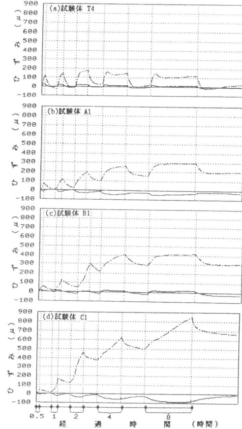
図14 試験体真ひずみの経時変化
