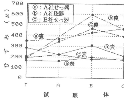
図13 最大実ひずみと下地積層との関係
