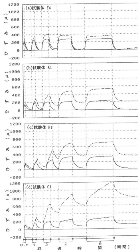
図8 タイル表裏の実ひずみの経時変化
