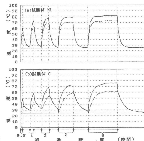
図3 試験体温度の経時変化
