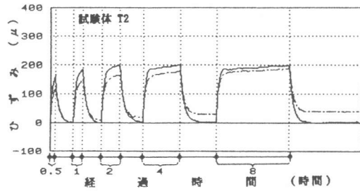
図5 試験体実ひずみの経時変化
