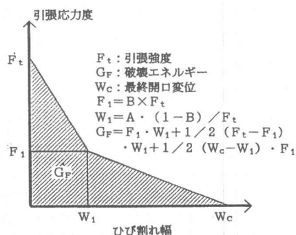
図-3 2直線引張軟化モデル
