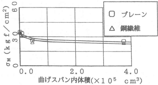
図-4 曲げ強度の寸法依存性
