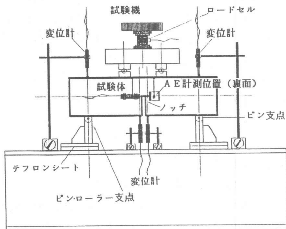
図-1 荷重方法
