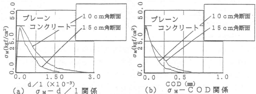
図-6 ノッチ入り試験体の荷重-変位関係
