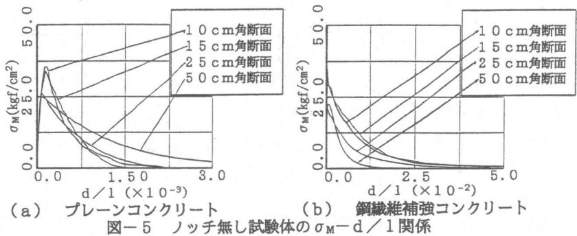
図-5 ノッチ無し試験体の \sigma_M-d/l 関係
