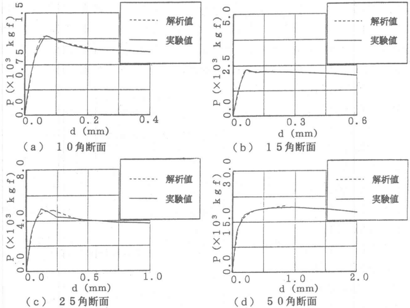
図-8 P-d 関係 (鋼繊維補強コンクリート)
