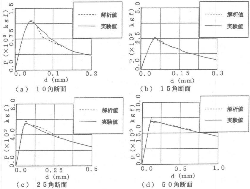
図-7 P-d 関係 (プレーンコンクリート)
