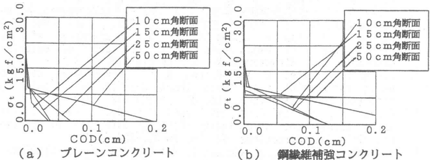
図-9 逆解析により得られた引張軟化特性
