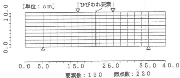
図-2 試験体のモデル化
