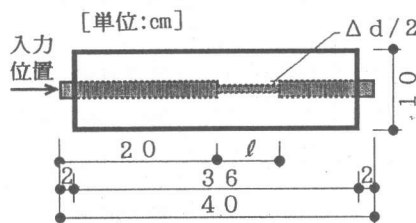
図-1 試験体の一例
