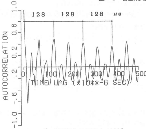
図-5 自己相関関数 (断面健全モデル)
