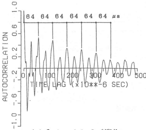
(a) \phi=4\text{cm} 、 \Delta d=8\text{mm} 試験体
