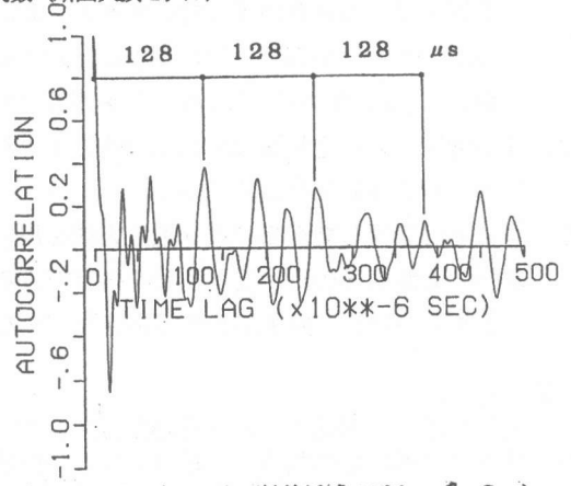
図-6 自己相関関数 (附着低減モデル、 \phi=8\text{cm} )
