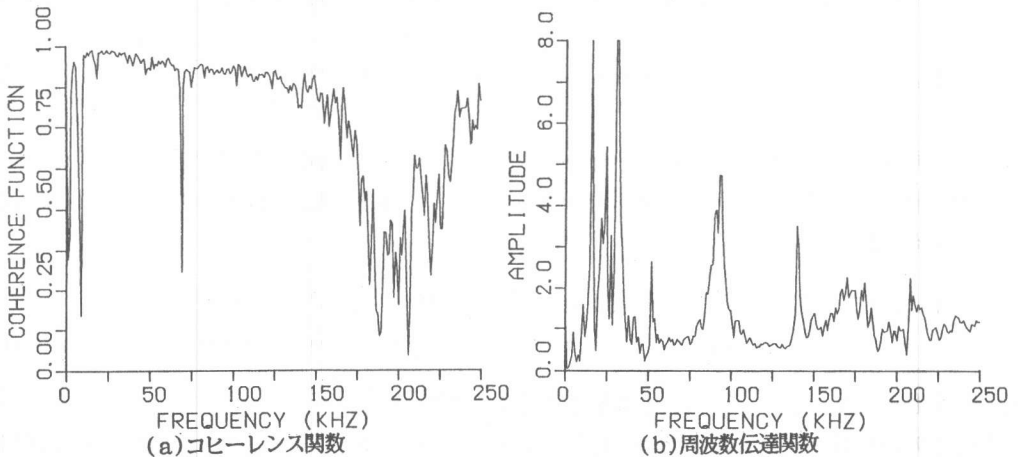
図-3 測定結果の周波数特性の一例 ( L=8 cm, \Delta d=8 mm)
