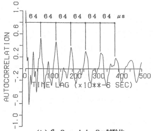
(b) \phi=8\text{cm} 、 \Delta d=8\text{mm} 試験体
