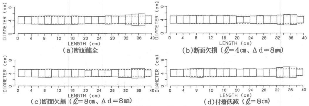
図-7 鉄筋断面の推定結果
