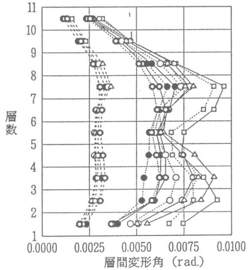
図6 最大層間変形角分布(50kine時)
