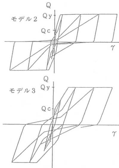
図2 接合部履歴モデル
