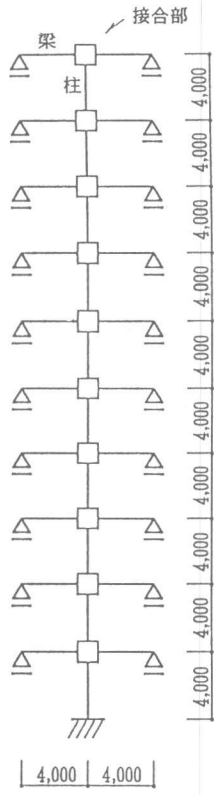
図1 モデル形状
