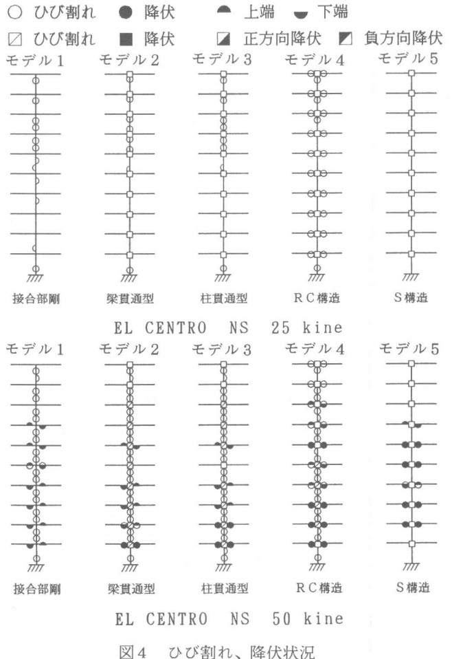
図4 ひび割れ、降伏状況
