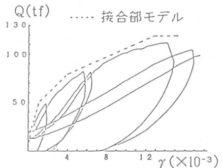
図3 実験結果との比較
