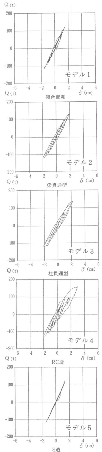
図8 層せん断力-層間変形関係
