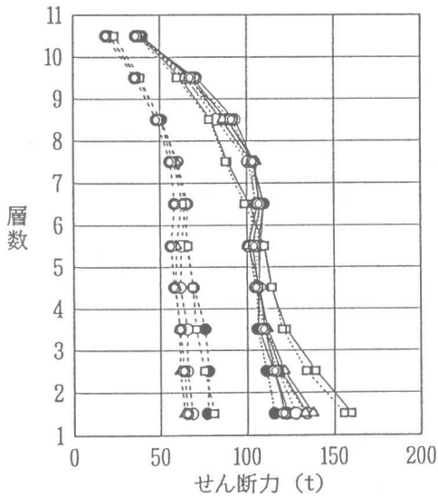
図5 最大層せん断力分布(50kine時)
