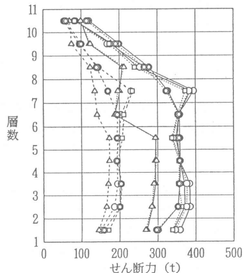
図7 接合部せん断力分布(50kine時)
