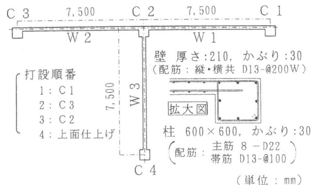
図-1 実大試験体の平面形状および配筋
