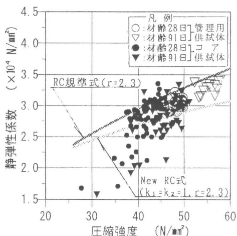
図-4 圧縮強度と静弾性係数の関係
