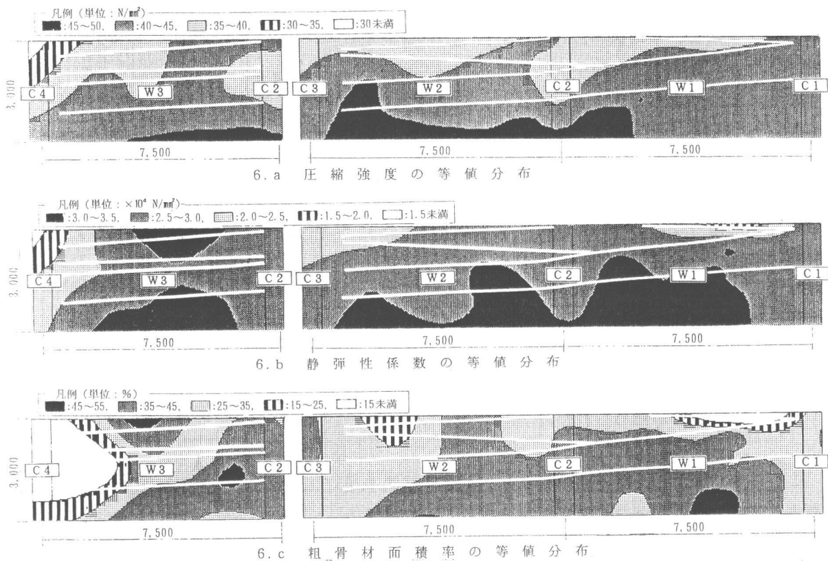
図一六 圧縮強度、静弾性係数および粗骨材面積率の等値分布[3] 註) 図中の白線は、打ち継ぎ位置における流動勾配を示す。
