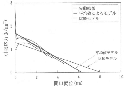
図-3 引張軟化曲線
