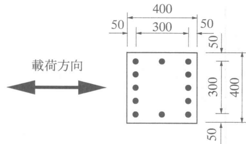
図－1 試験体柱部断面
