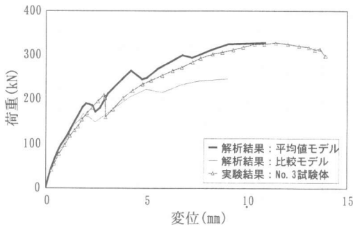
図-4 引張軟化曲線による解析結果の相違
