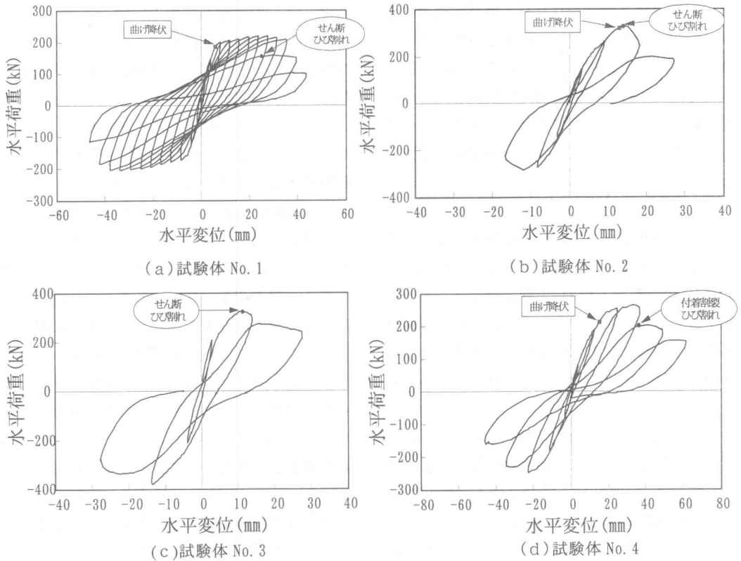
図-2 交番載荷実験結果：荷重-変位曲線
