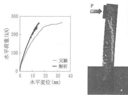
図-5 解析結果：No.4試験体
