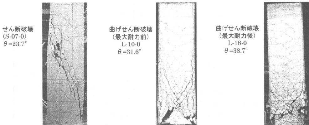
写真-1 試験体終局ひび割れ状況
