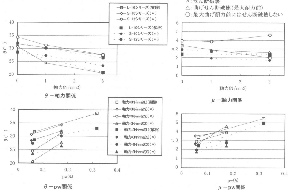
図-3 実験および解析結果比較
