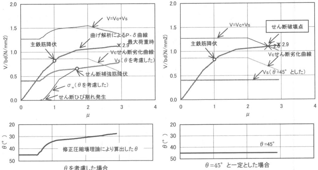
図-4 評価例(S-15-0)
