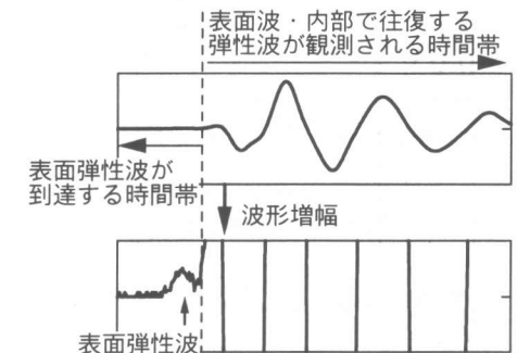
図-5 測定波形の増幅による表面弾性波の観測
