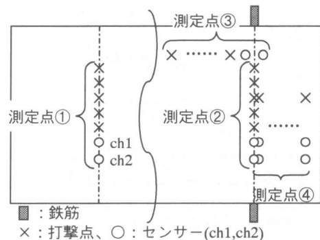
図-6 内部鉄筋の影響調査実験状況
