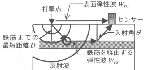
図-9 弾性波の伝搬モデル
