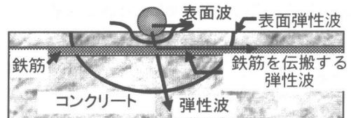
図-1 コンクリートに発生する振動
