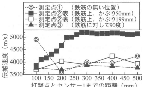
図-7 伝搬速度と打撃点位置の関係
