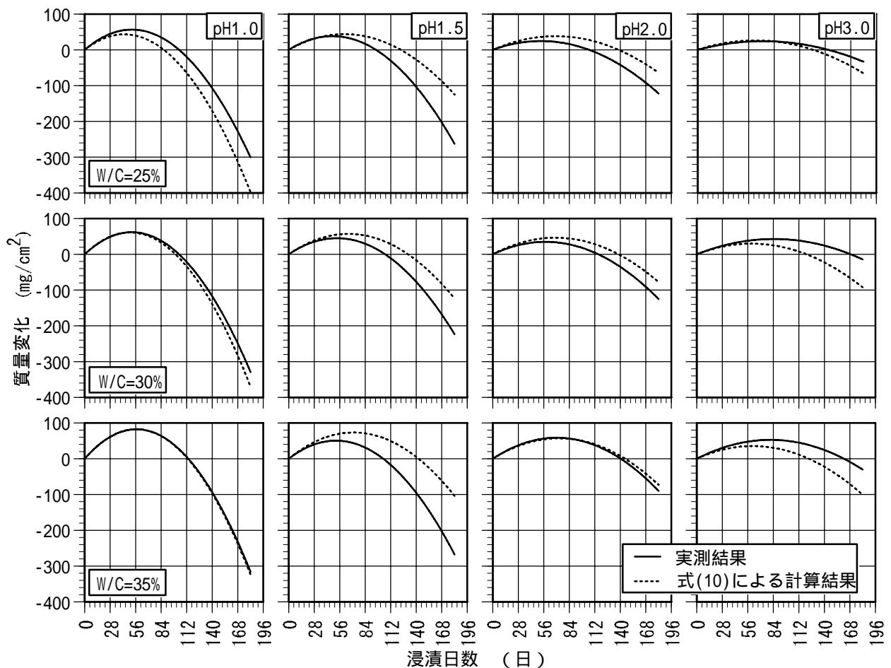
図 - 5 内側暴露試験体の経時変化の比較
