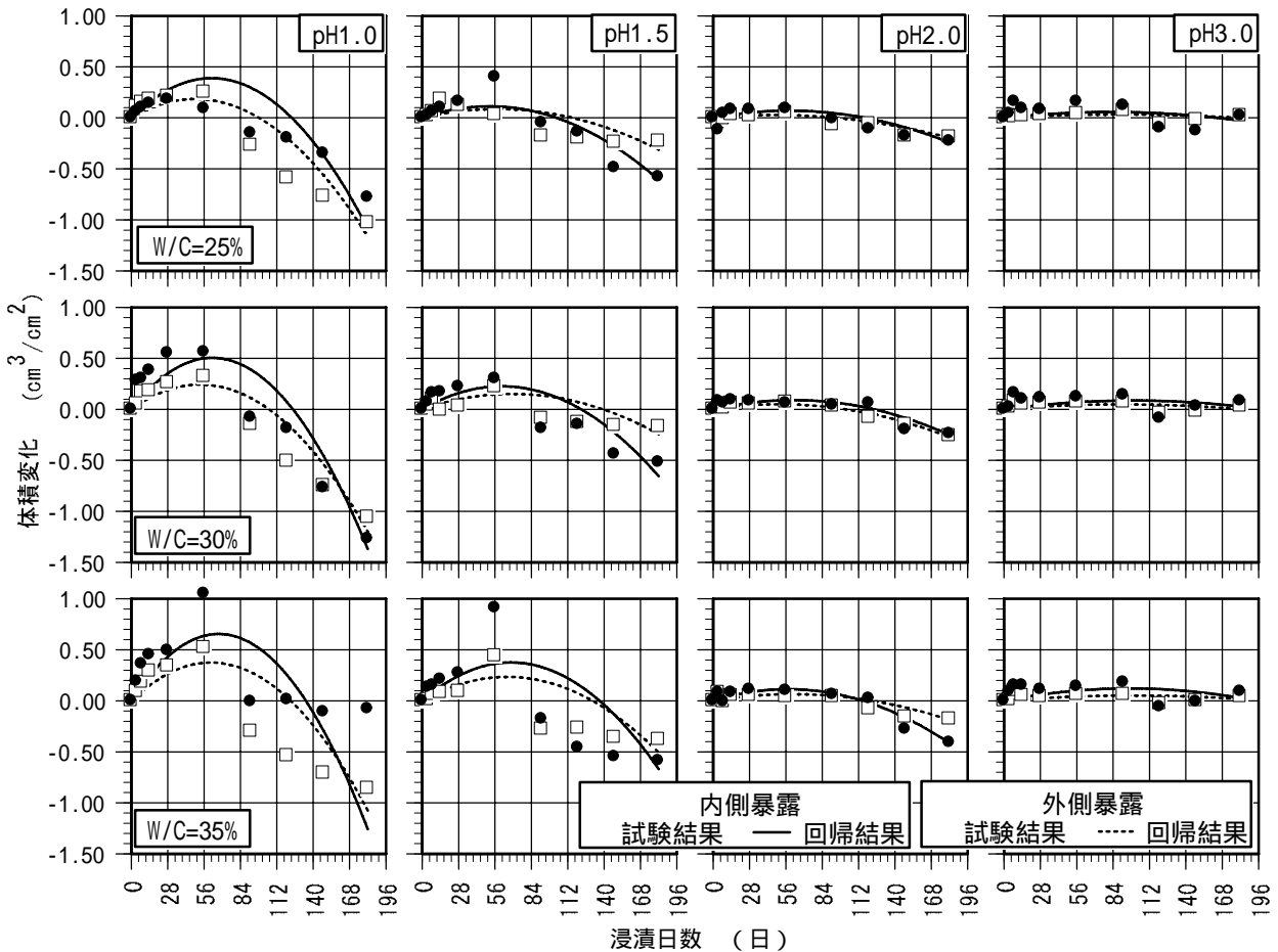
図 - 4 浸漬日数と表面積当りの体積変化
