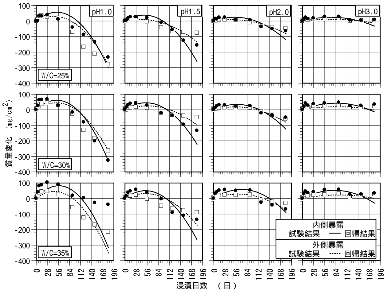
図 - 3 浸漬日数と表面積当りの質量変化
