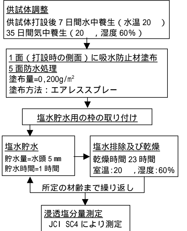
図-1 塩分浸透試験フロー
