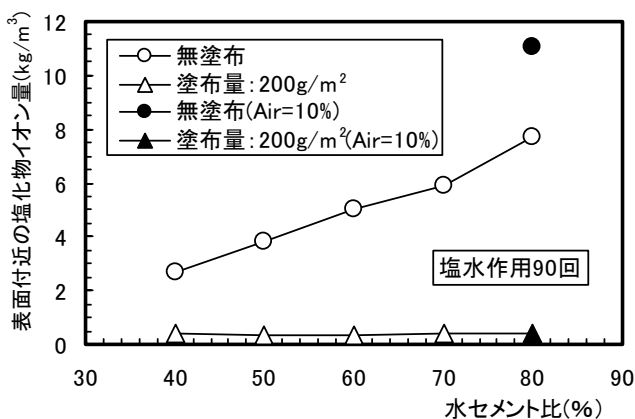
図-6 水セメント比と塩化物イオン量の関係
