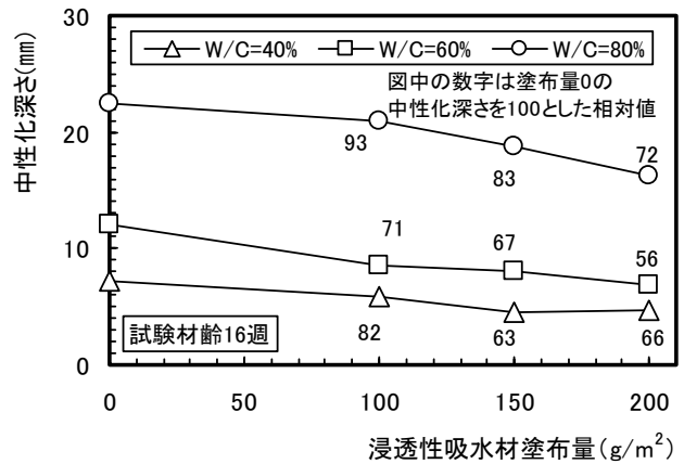
図-10 吸水防止材塗布量と中性化深さの関係
