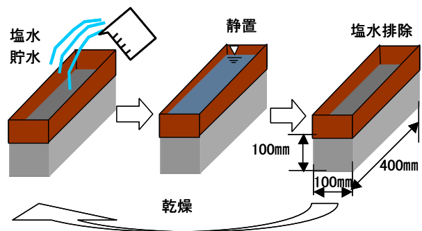
図-2 塩分浸透試験概略図
