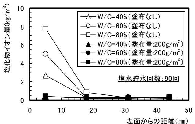
図-5 塩化物イオンの浸透状況(塩水作用90回)
