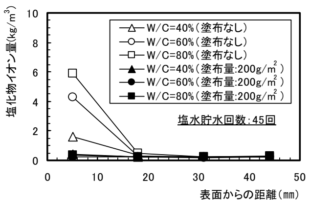
図-4 塩化物イオンの浸透状況(塩水作用45回)
