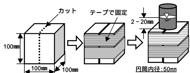
図-3 ひび割れ透水試験供試体作製方法
