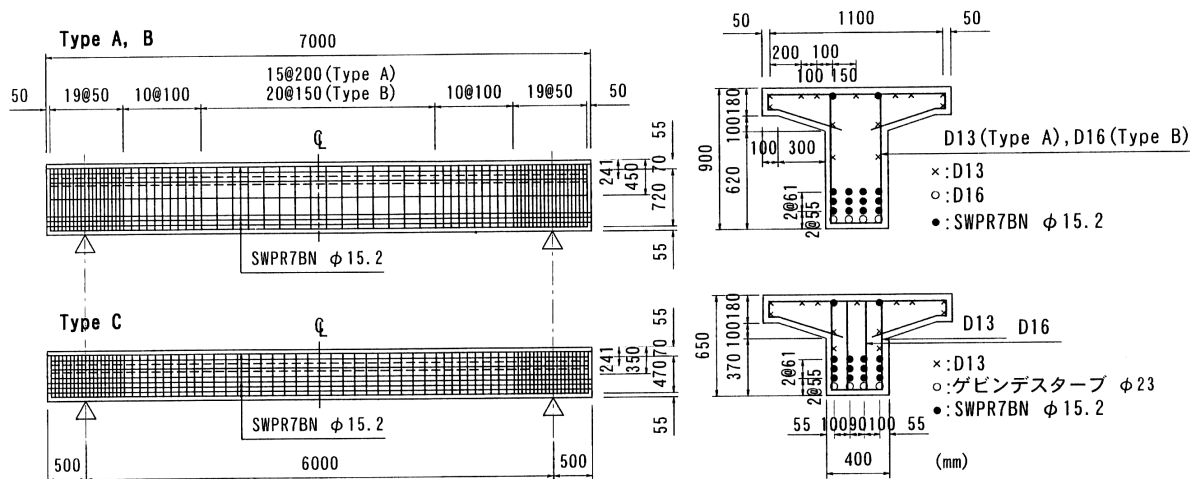
図 - 1 試験体の形状寸法および配筋図
