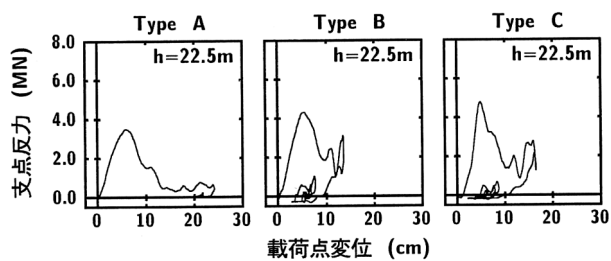
図 - 2 支点反力 - 载荷点変位履歴曲線
