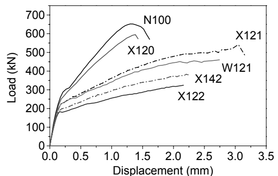
図-7 荷重変位関係(解析値)
