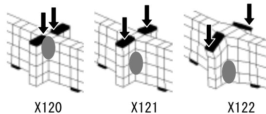
図-9 横梁から梁本体へのせん断力伝達位置 （●がせん断力伝達位置の中心）
