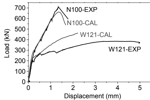
図-10 荷重変位関係（実験と解析）
