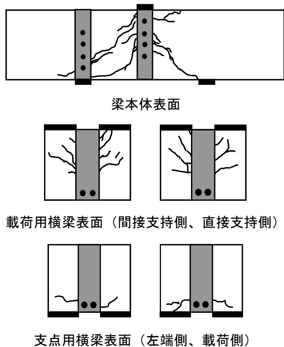
図-11 ひび割れ図 W121-EXP (破壊時)
