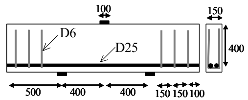
図-1a 供試体概要図 N100
