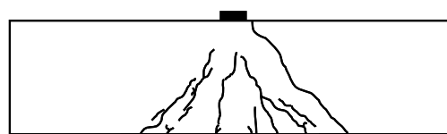
図-5a ひび割れ図 N100-EXP (破壊時)
