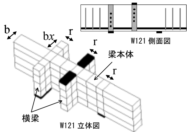
図-2 試験体 W121 概要図 (黒色部分は載荷板)
