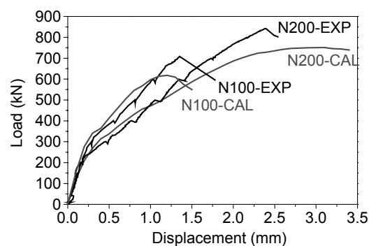
図-4 実験および解析結果
