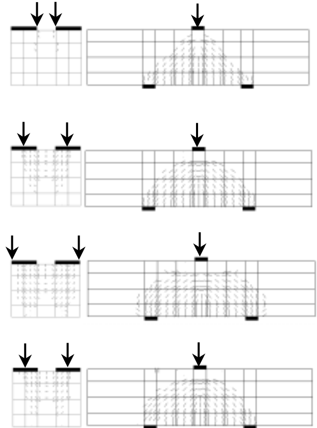
図-8 ひび割れ図（横梁および梁本体の中央） 上から X120、X121、X122、W121（300kN時）
