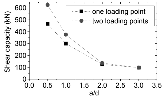
図-6 a/dによる荷重点数の影響の違い(解析)
