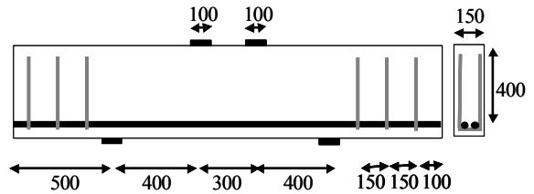
図-1b 供試体概要図 N200
