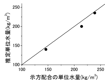
図-5 単位水量の推定結果
