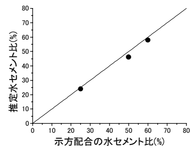
図-3 水セメント比の推定結果
