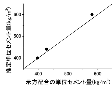
図-4 単位セメント量の推定結果
