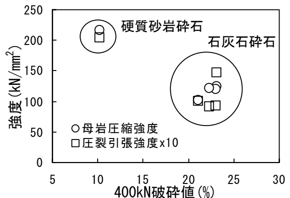
図-1 400kN 破砕値と骨材強度の関係
