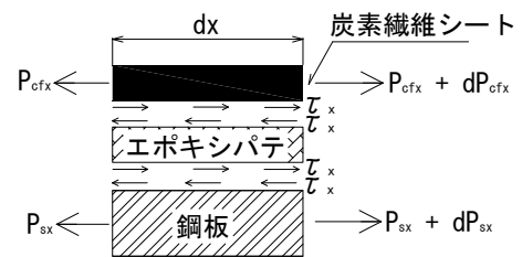
図-8 微小要素の力釣り合い図
