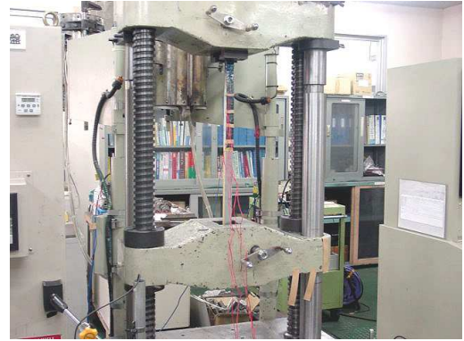
写真-1 試験機および試験体設置状況
