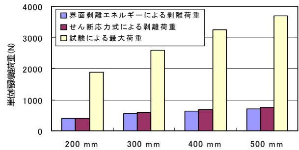
図-9 剥離荷重計算と実験の最大荷重
