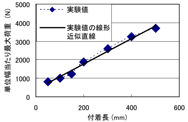
図-6 単位幅当たり最大荷重-付着長の関係
