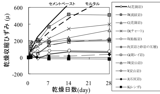
図-7 骨材コアの乾燥収縮の経時変化
