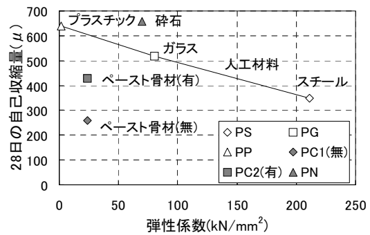
図-4 自己収縮量-骨材弾性係数関係
