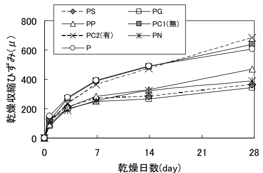
図-5 乾燥収縮の経時変化
