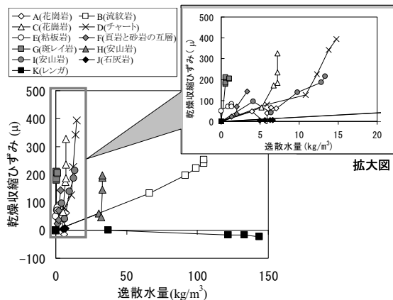
図-8 乾燥収縮ひずみ-水分逸散量関係
