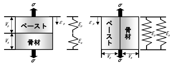
a)完全直列複合則 b)完全並列複合則
