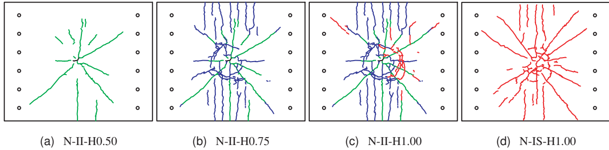
図-7 RCスラブ下面のひび割れ状況
