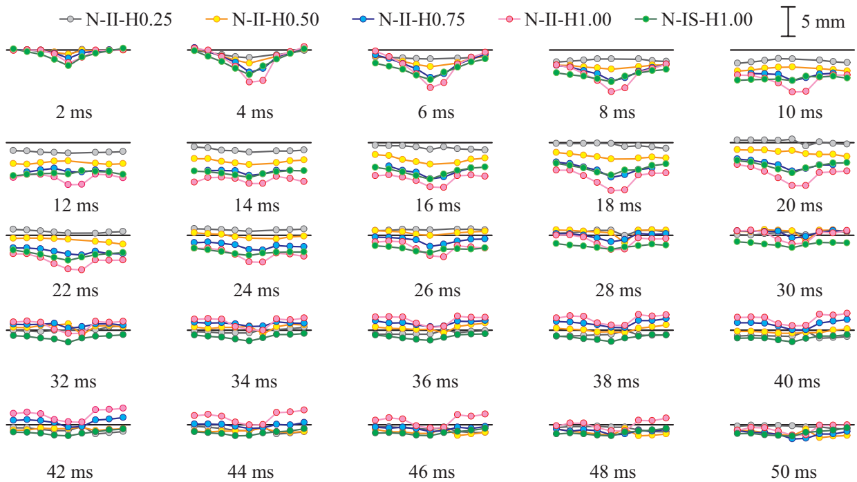
図-5 スパン直角方向変位分布
