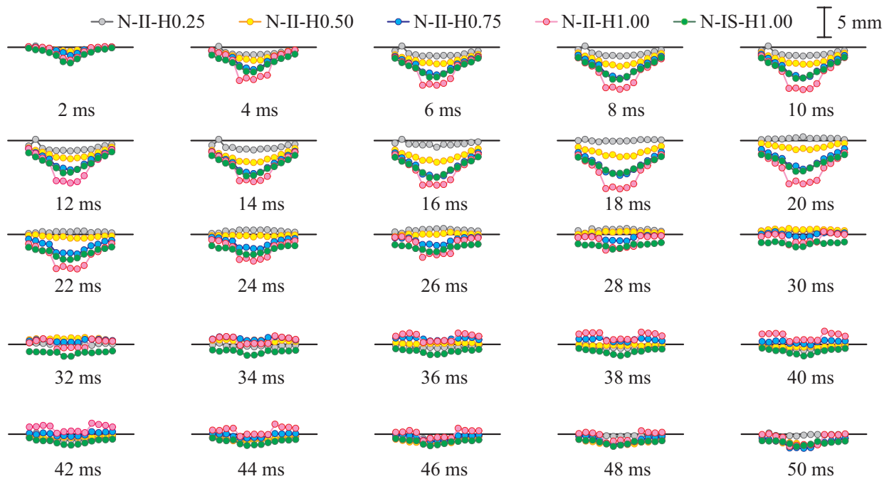
図-4 スパン方向変位分布
