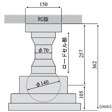
図-3 隅角点支持部の状況
