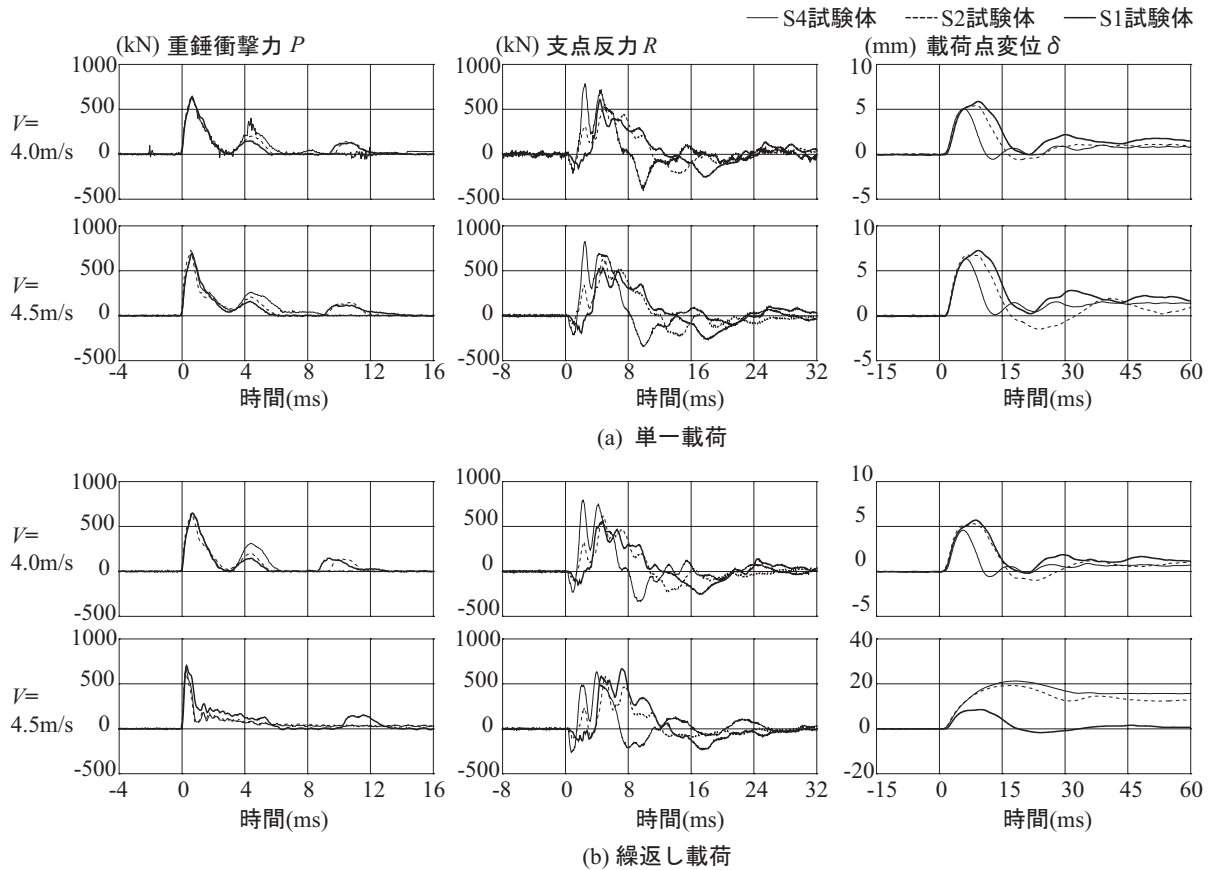
図-5 重錘衝撃力、支点反力および载荷点変位に関する応答波形
