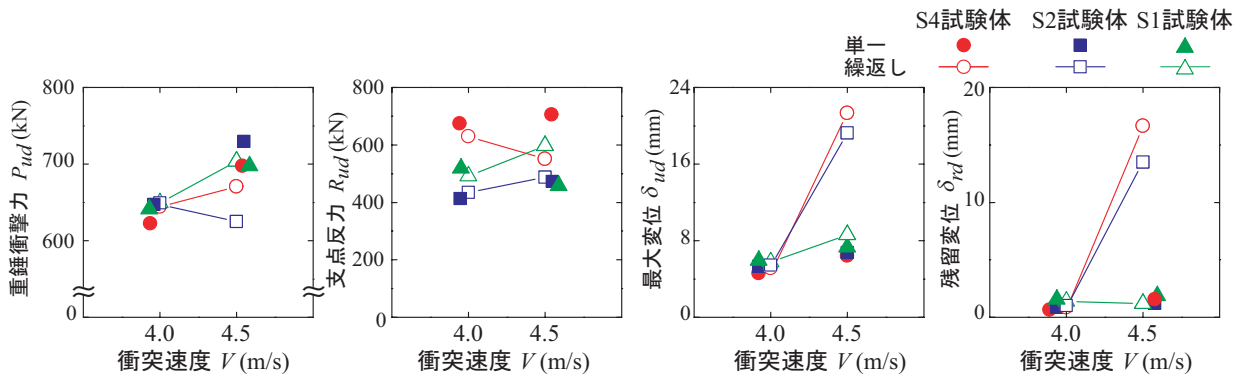
図-6 重錘衝撃力、支点反力、最大および残留変位と衝突速度との関係
