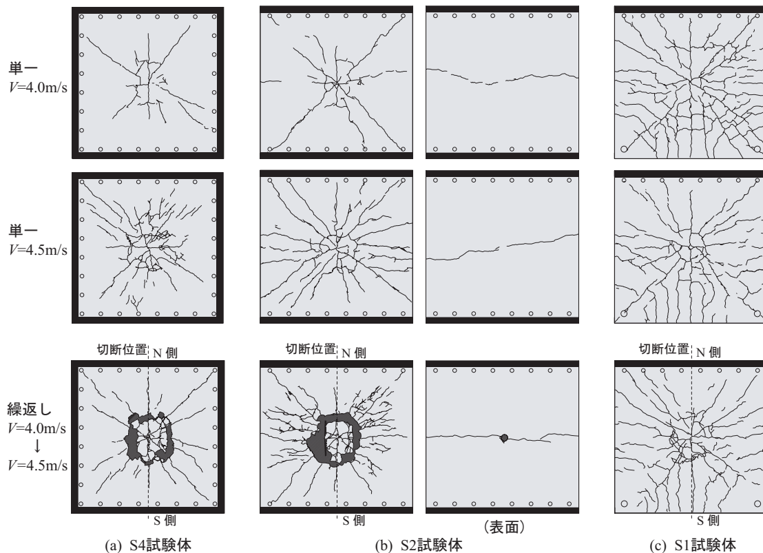
図-4 実験終了後におけるRC版裏面のひび割れ分布性状
