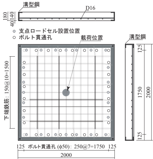
(a) 四辺支持
