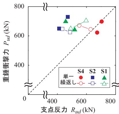
図-7 重錘衝撃力と支点反力との関係
