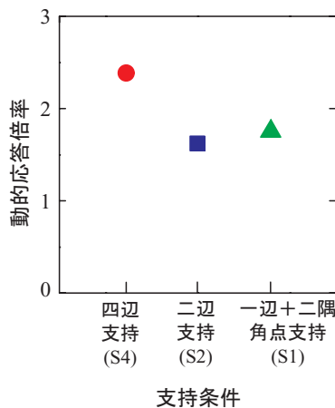
図-8 動的応答倍率
