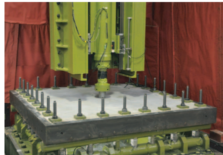
(a) 四辺支持
