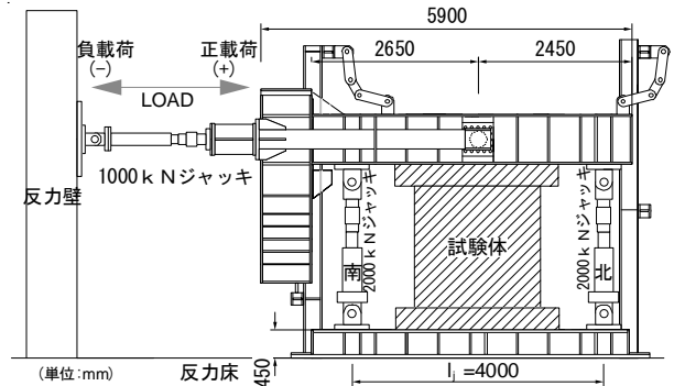
図-3 荷重装置
