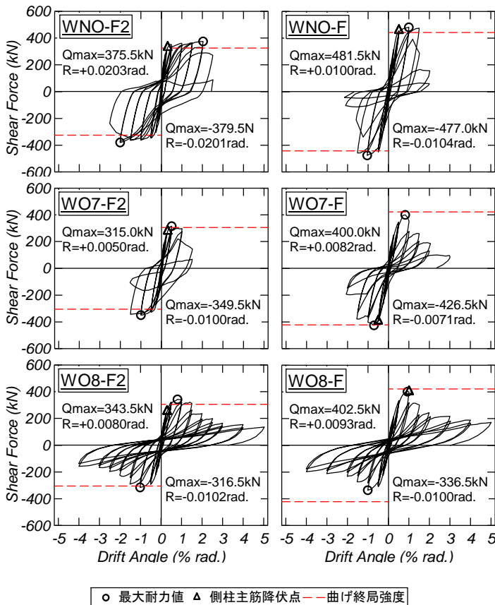
図-5 せん断力-変形角関係 (上図：本実験 下図：2010年度実験)
