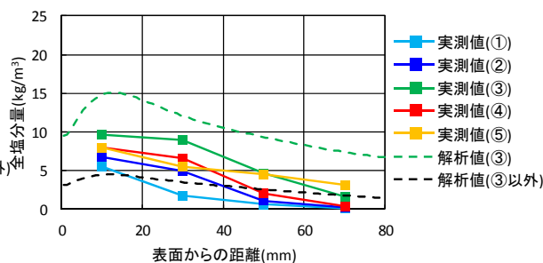
図-18 B橋塩分浸透量比較
