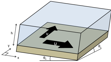
図-2 構造物表面における水の流れ
