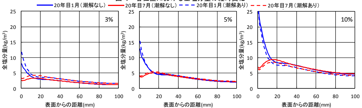
図-10 全塩分量の分布の経時変化
