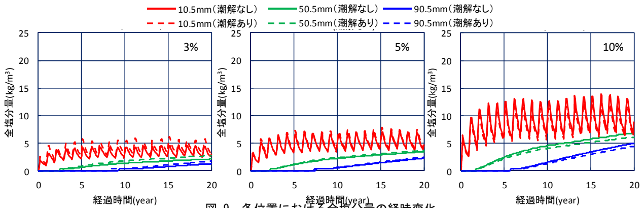
図-9 各位置における全塩分量の経時変化
