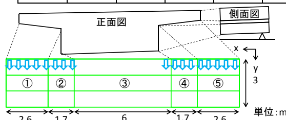
図-13 B橋模式図
