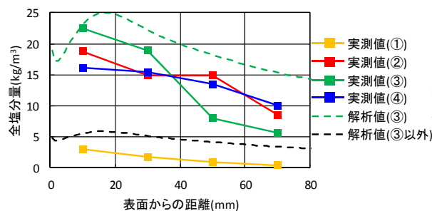
図-17 A橋塩分浸透量比較
