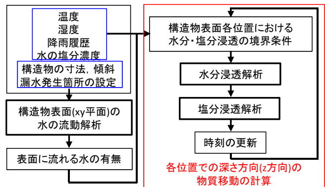
図-1 解析全体概要
