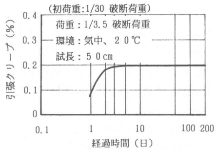
図-2 クリープ試験結果
