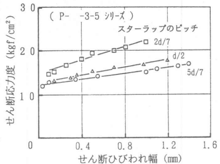
図-6 せん断応力度とせん断ひびわれ幅の関係
