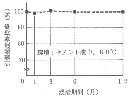
図-1 耐アルカリ性試験結果
