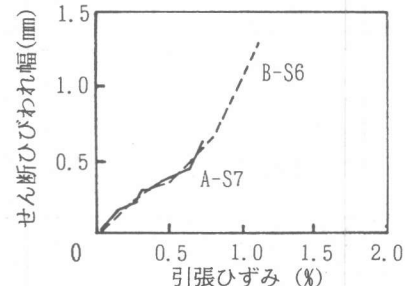
図-9 せん断ひびわれ幅とスターラップのひずみの関係
