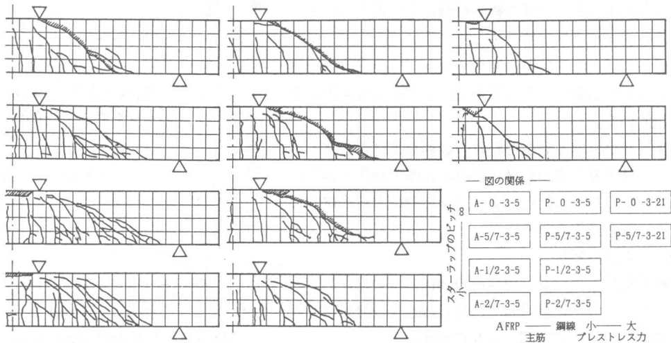
図-5 ひびわれ状況
