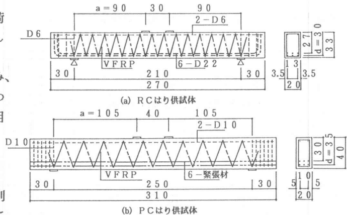
図-4 供試体配筋図(単位;cm)
