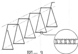
図-3 せん断補強用VFRPロッド概要図
