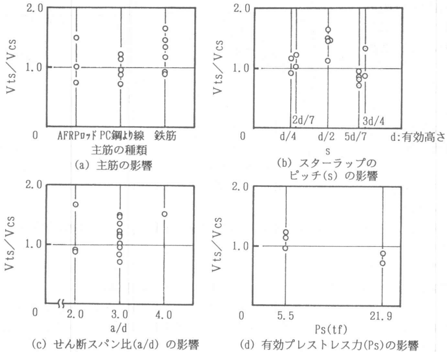
図-1 1 スターラップの効果に関する計算値と実験値の比較
