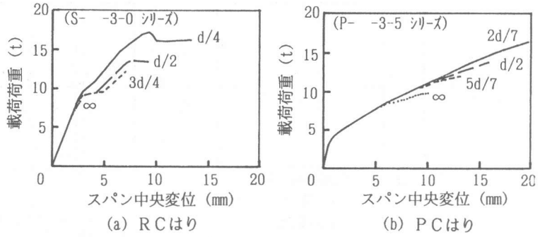
図-10 載荷荷重とスパン中央変位の関係
