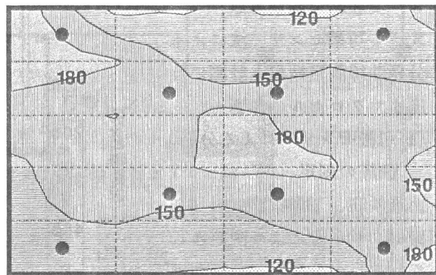
単位: mV ●: 電極挿入位置
