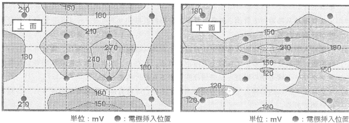
図-8 通電2時間後分極量等電位線 (マクロセル系, 下部挿入型電極10本, 12.5mA)
