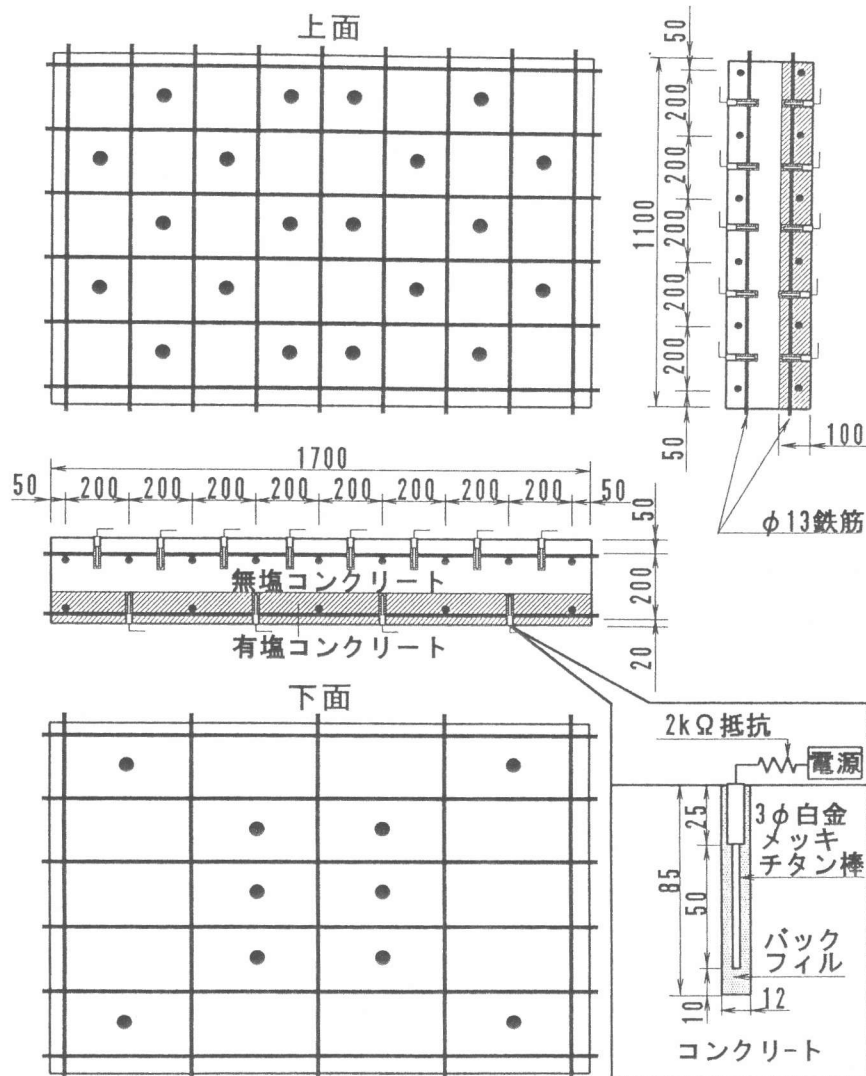
図-1 コンクリート供試体及び供試電極位置（●：電極挿入位置）
