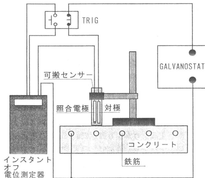
図-2 可搬センサー法による分極曲線測定装置
