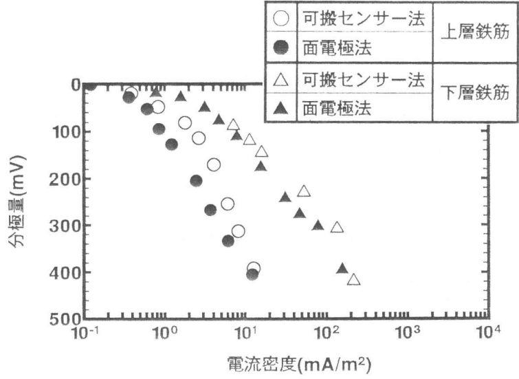
図-4 可搬センサー法と面電極法による鉄筋の分極曲線
