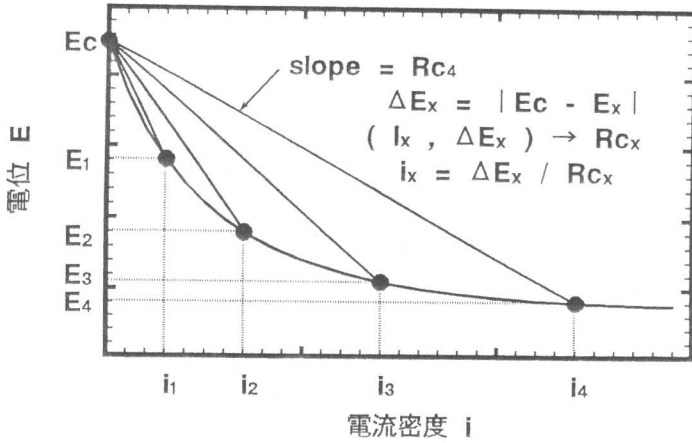
図-3 可搬センサー法からの電流密度の算出
