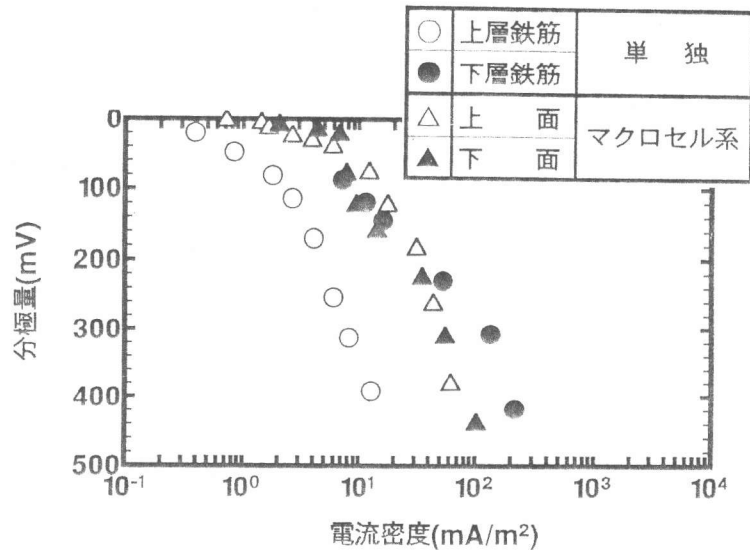
図-5 マクロセル系における鉄筋の分極曲線 (可搬センサー法)
