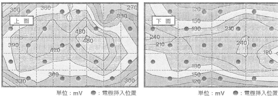
図-9 通電2時間後分極量等電位線 (マクロセル系, 上部挿入型電極20本, 25.0mA)
