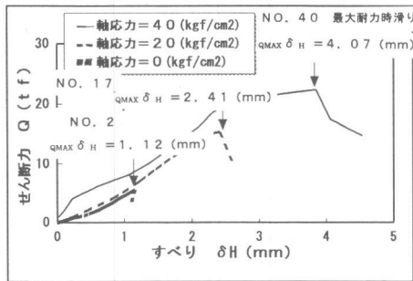
図15 R_z がほぼ等しく軸力の異なる 3試験体の Q_{max} - \delta H 関係
