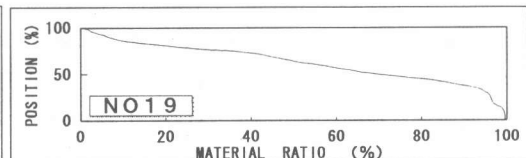
図7 負荷曲線
