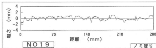
図6 粗さ曲線
