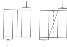
図8 滑り破壊 図9 せん断破壊
