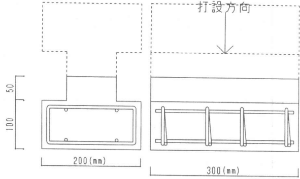
図1 試験体断面
