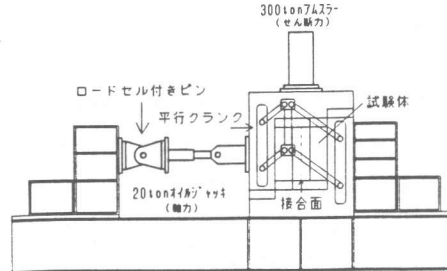
図5 載荷装置
