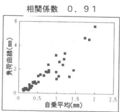
図 14 粗さ相関関係
