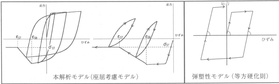
図4 鋼管の応力-ひずみ関係
