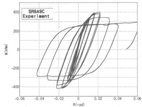
図7 材端モーメント(M)－一部材角(R)関係の比較 (SR6C4C, SR6A9C 試験体、CASE1 と同様の解析モデル)
