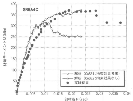
図 5 材端モーメント (M) - 部材角 (R) 関係の比較 (拘束効果考慮の有無による比較: SR6A4C 試験体)
