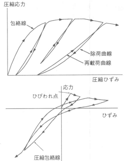
図3 コンクリートの応力-等価一軸ひずみ関係
