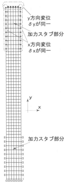
図2 要素分割
