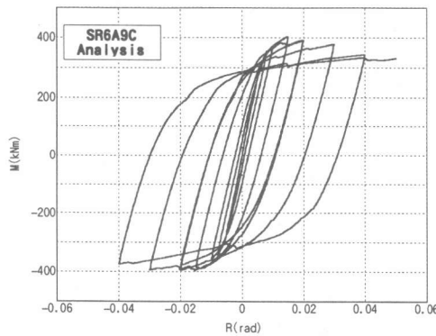
図7 材端モーメント(M)－一部材角(R)関係の比較 (SR6C4C, SR6A9C 試験体、CASE1 と同様の解析モデル)
