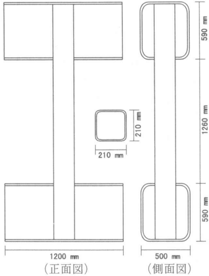
図1 試験体形状
