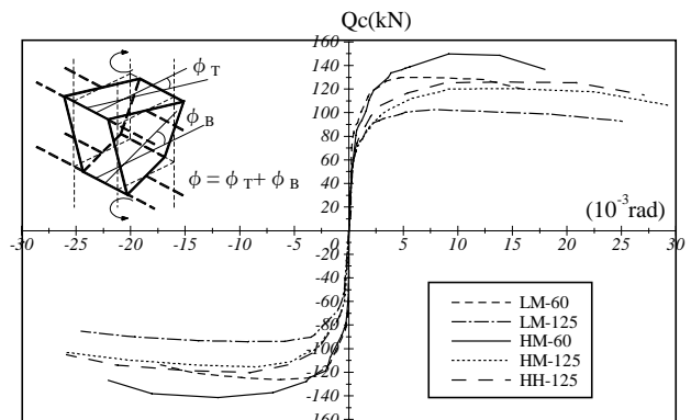
図-4 層せん断力-接合部捩れ変形角関係
