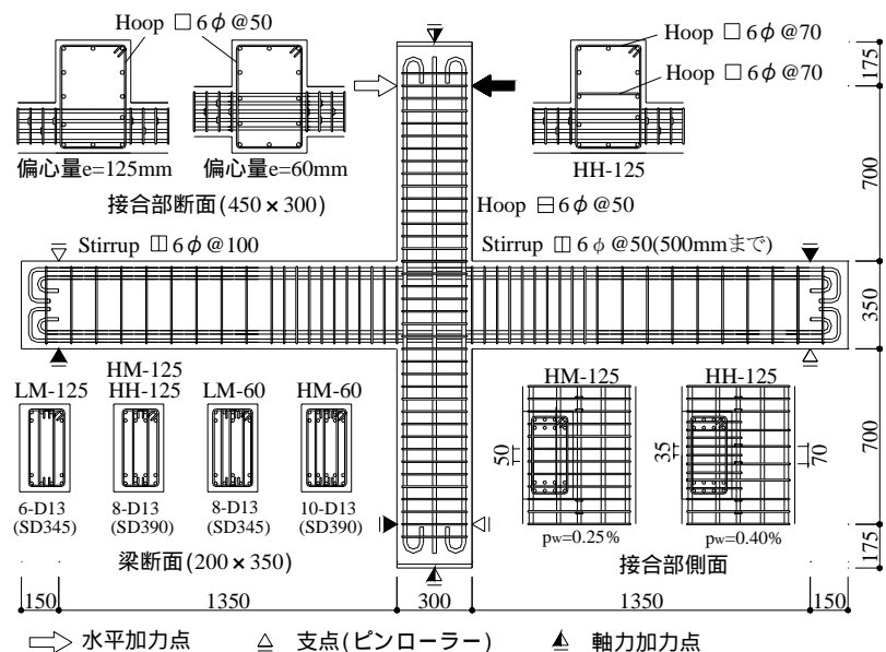
図-1 試験体概要 (単位 mm)
