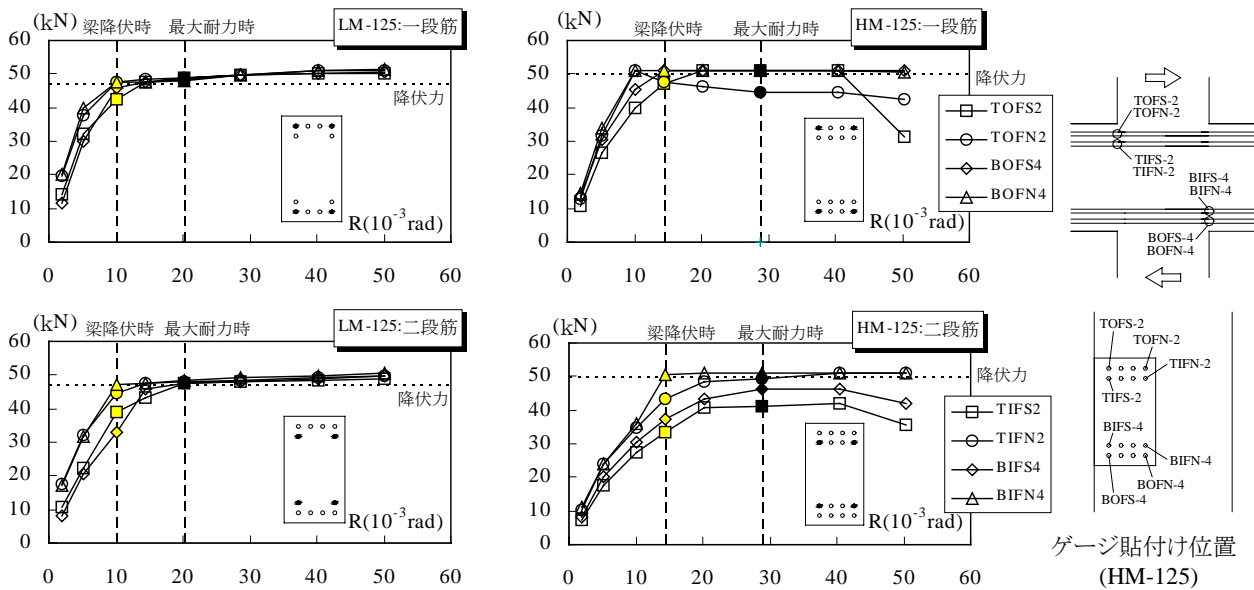
図-6 梁主筋応力の推移
