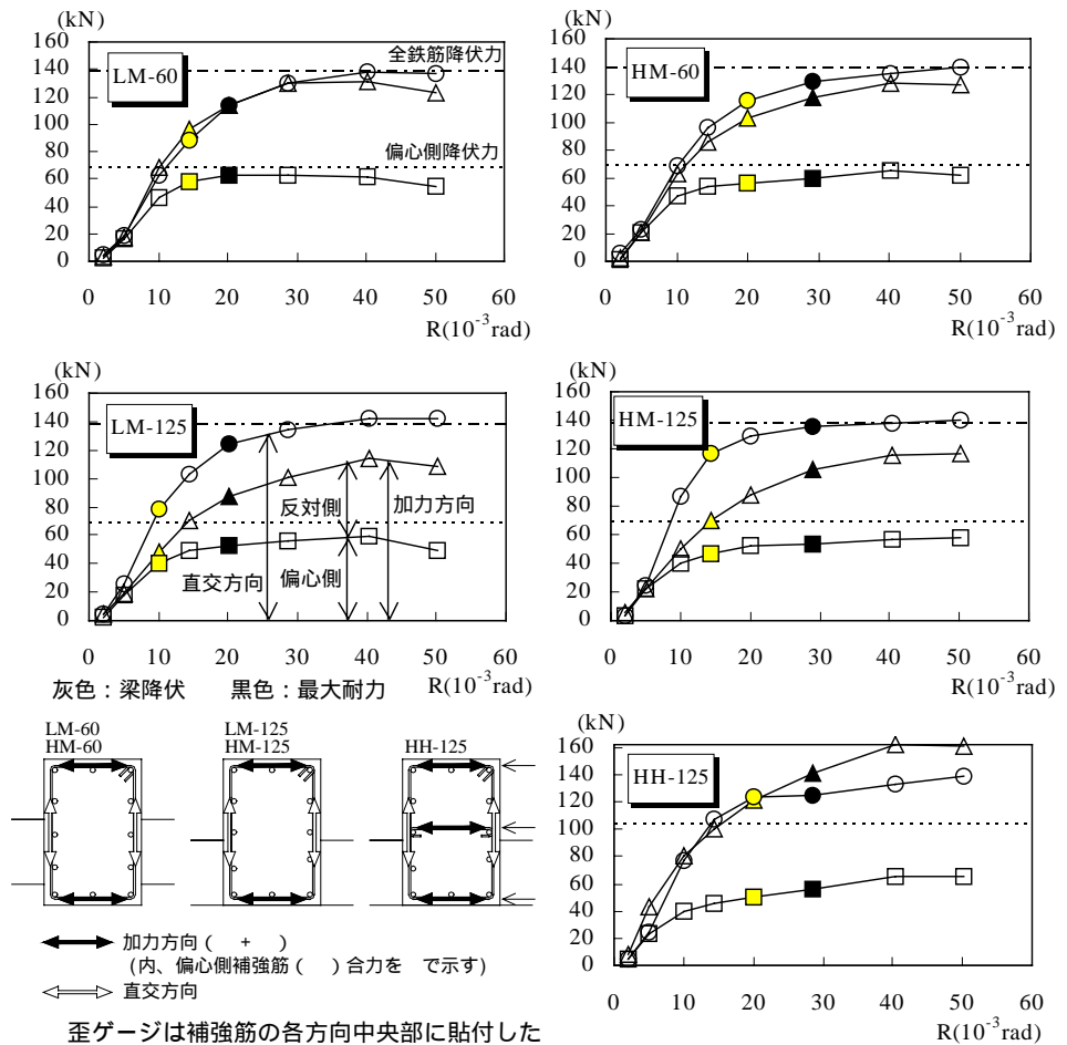
図-7 接合部補強筋合力の推移
