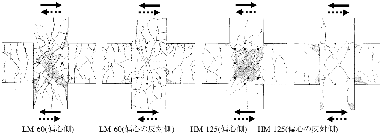
図-2 最終破壊状況 (ハッチはカバーコンクリートの剥落を表す)
