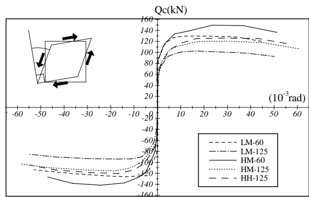
図-5 層せん断力-接合部せん断変形角関係
