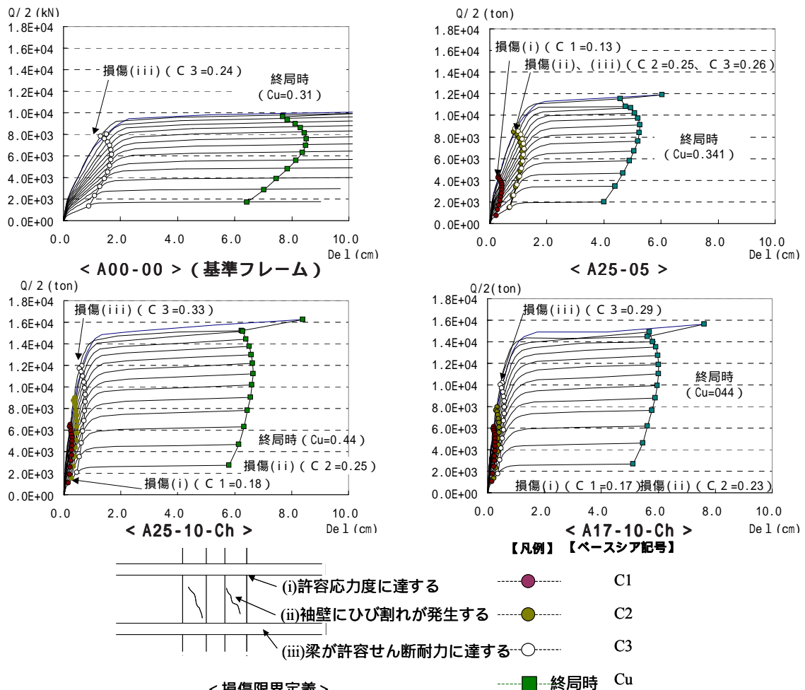
図-4 層せん断力-層間変位関係
