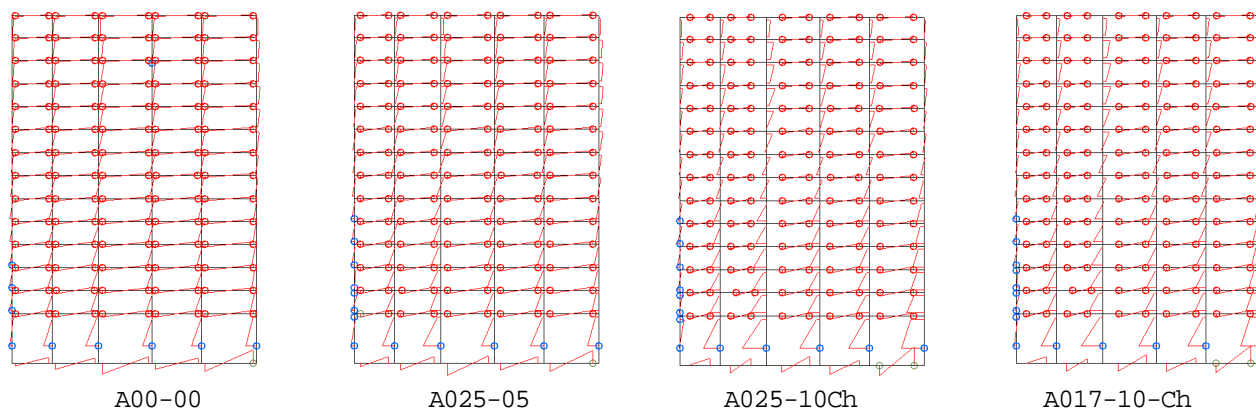
図 - 5 終局時モーメント分布比較 (○はヒンジを示す)
