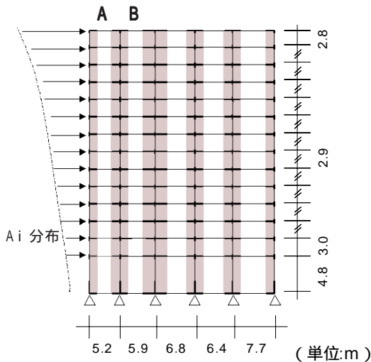
図-3 フレーム形状及び加力方式
