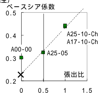
図-7 ベースシア係数 - 張出比関係 (終局時)
