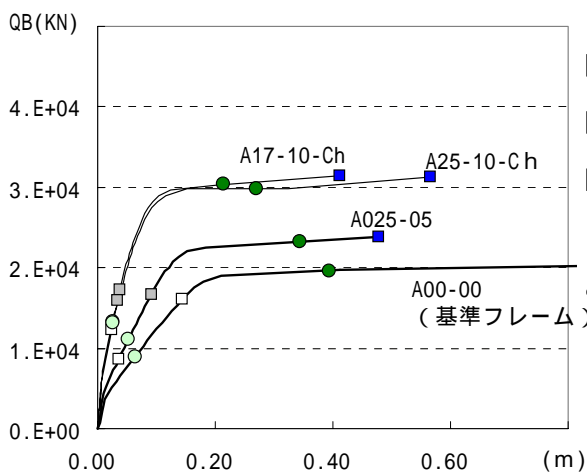
図-6 ベースシア - 代表変位関係
