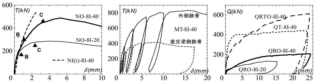
図 - 3 荷重 - 変形関係 (包絡線)
