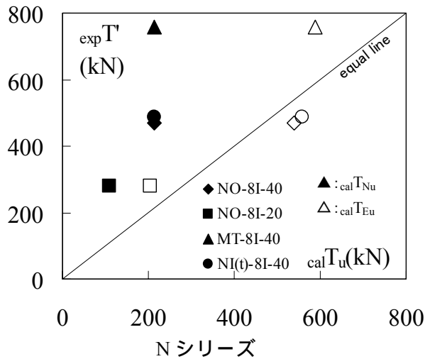
図 - 4 実験値と計算値の耐力比較
