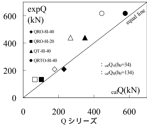
図 - 4 実験値と計算値の耐力比較
