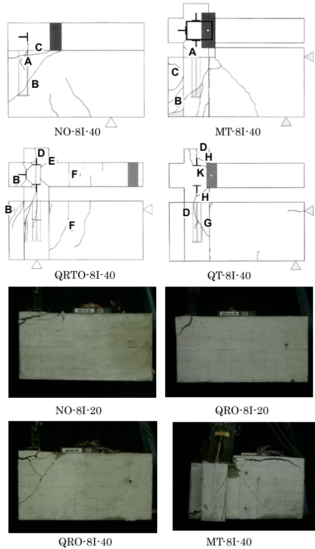
図 - 2 亀裂図
