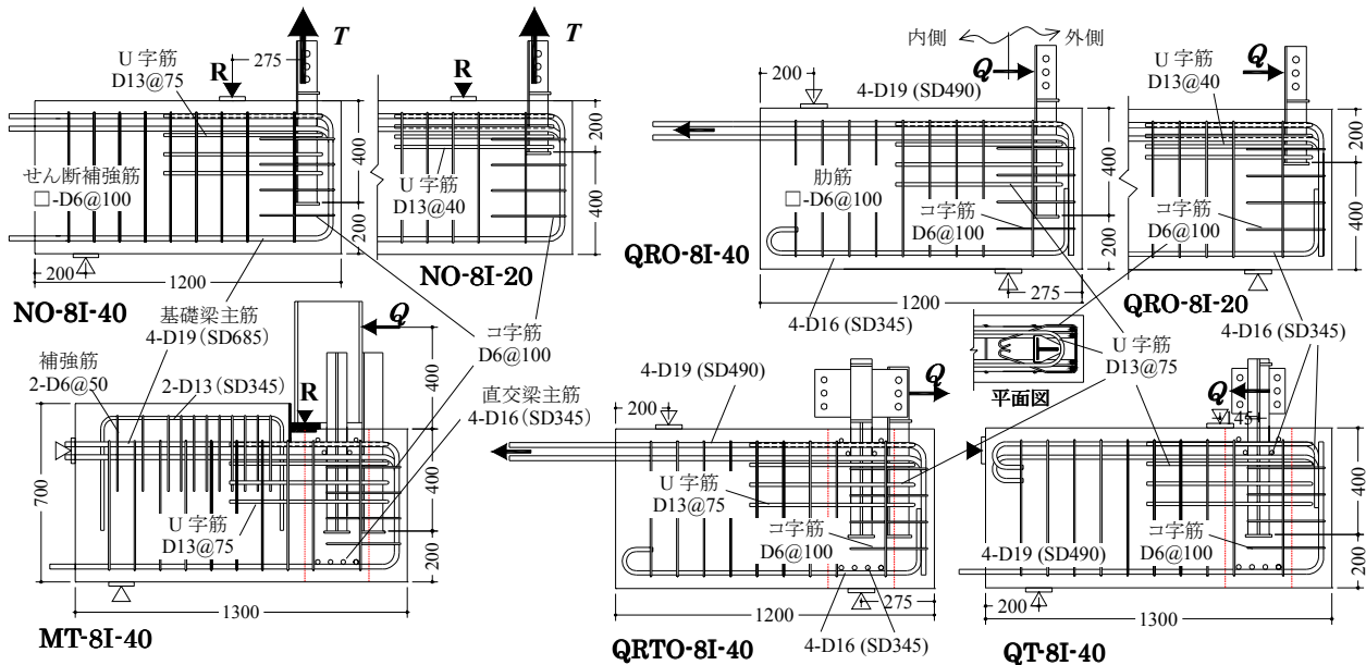
図 - 1 試験体形状
