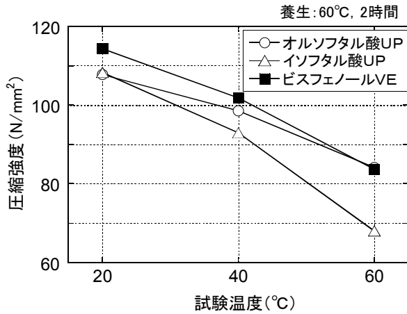
図 - 1 試験温度と圧縮強度
