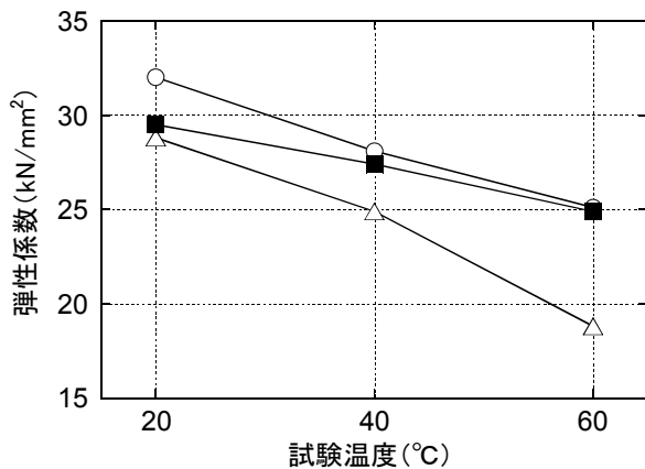
図 - 3 試験温度と弾性係数
