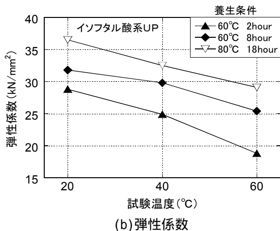
図 - 6 試験温度と物性(養生温度)
