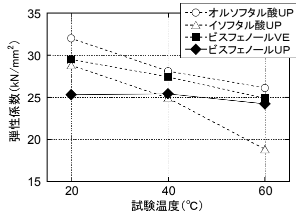
図 - 10 試験温度と弾性係数
