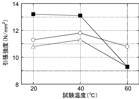
図 - 2 試験温度と引張強度
