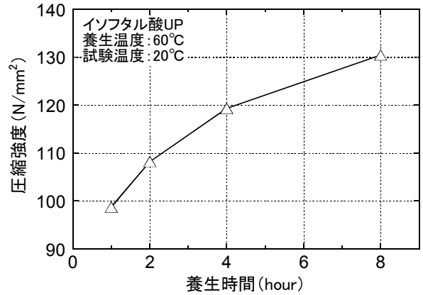
図 - 4 養生時間と圧縮強度
