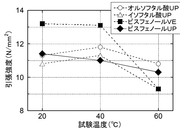
図 - 9 試験温度と引張強度
