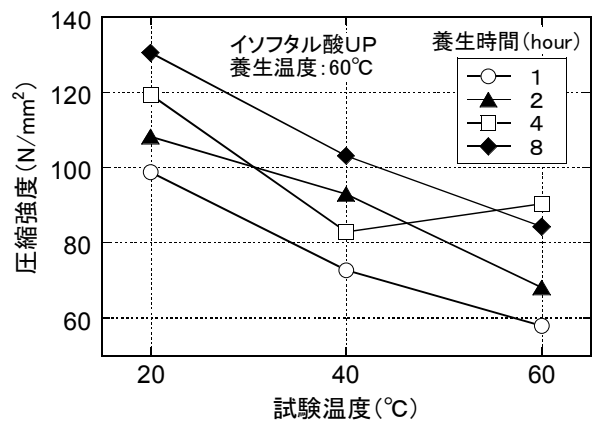
(a) 圧縮強度
