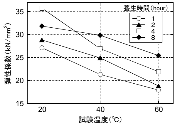
(b) 弾性係数
