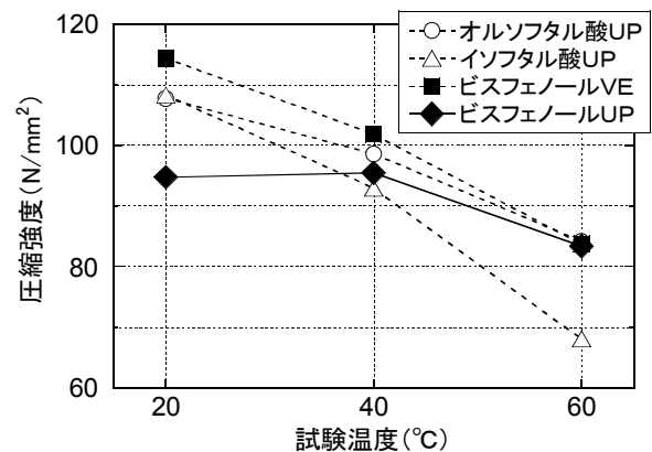
図 - 8 試験温度と圧縮強度
