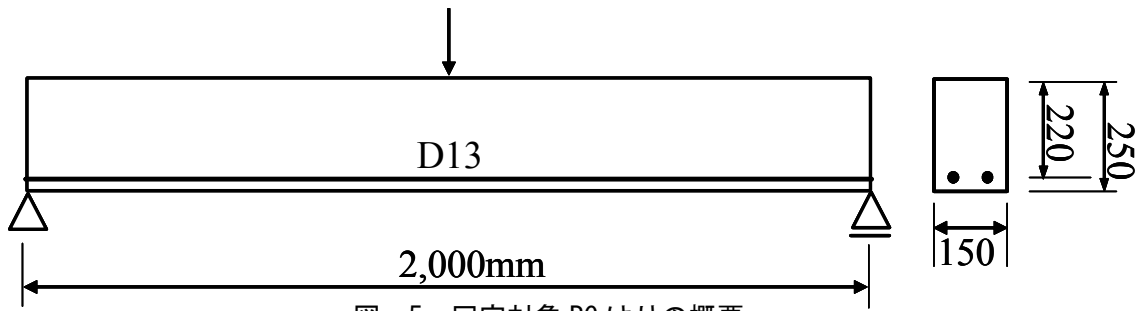
図-5 同定対象 RC はりの概要
