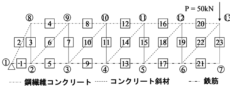
図-6 RC はりのトラスモデル図
