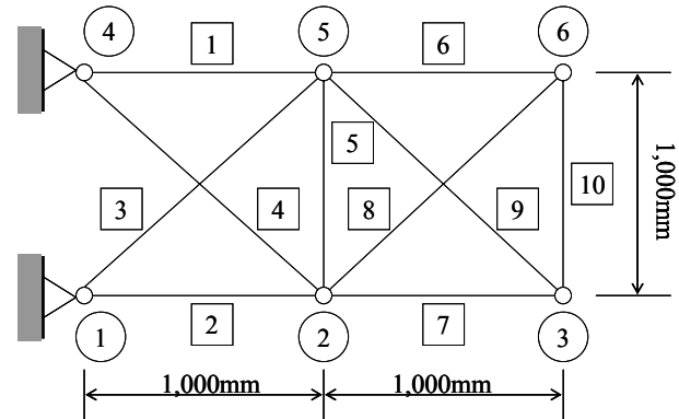
図-3 10 部材トラス構造物
