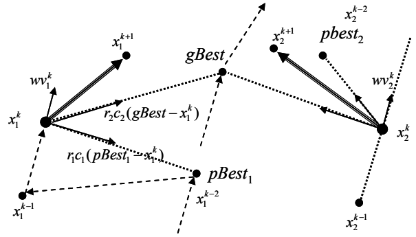
図-1 移動する粒子の模式図
