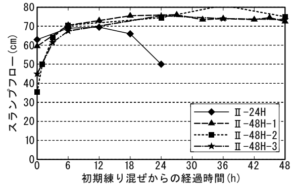
図-5 スランプフローの経時変化 (シリーズII初期練り混ぜ以降)
