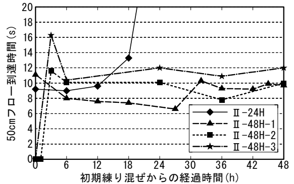
図-6 50cm フロー到達時間の経時変化 (シリーズII初期練り混ぜ以降)
