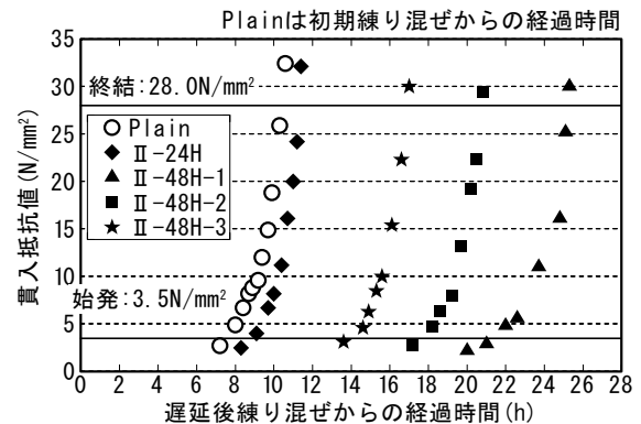
図-11 遅延後練り混ぜ以降の凝結性状
