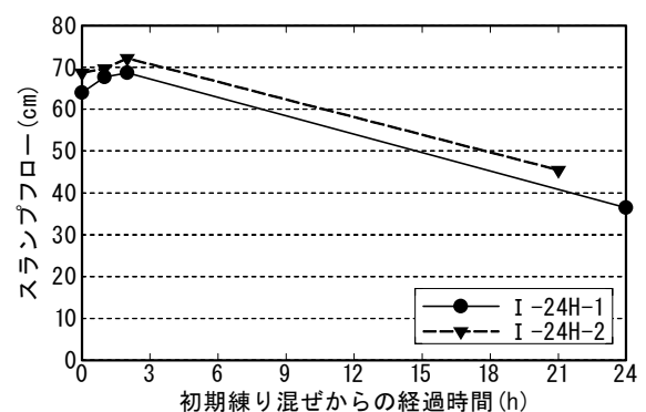
図-2 スランプフローの経時変化 (シリーズ I 初期練り混ぜ以降)
