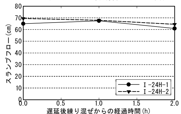
図-3 スランプフローの経時変化 (シリーズ I 遅延後練り混ぜ以降)
