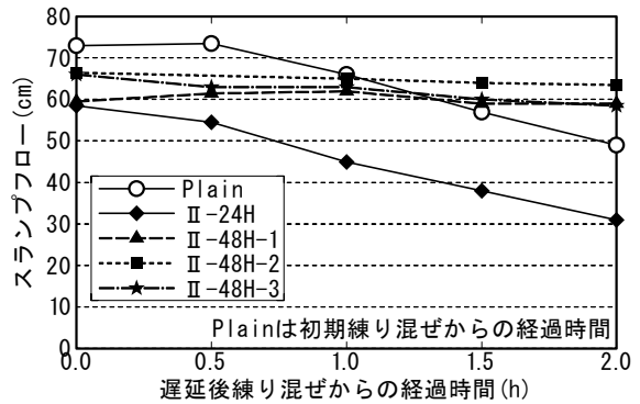
図-7 スランプフローの経時変化 (シリーズII遅延後練り混ぜ以降)
