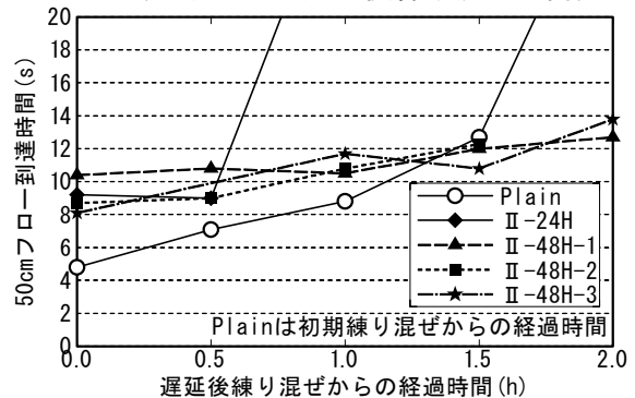
図-8 50cm フロー到達時間の経時変化 (シリーズII遅延後練り混ぜ以降)
