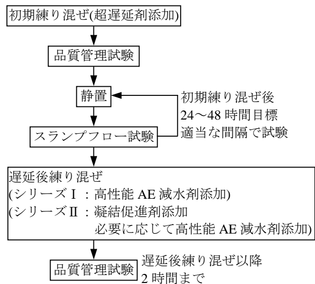
図-1 凝結時間制御フロー
