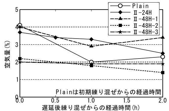
図-9 空気量の経時変化 (シリーズ II 遅延後練り混ぜ以降)
