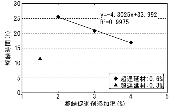
図-12 凝結促進剤の添加量 と凝結時間の比較
