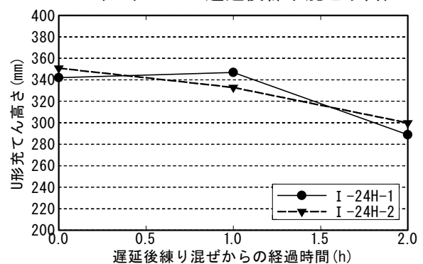
図-4 U形充てん高さの経時変化 (シリーズ I 遅延後練り混ぜ以降)
