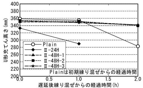
図-10 U 形充てん高さの経時変化 (シリーズ II 遅延後練り混ぜ以降)
