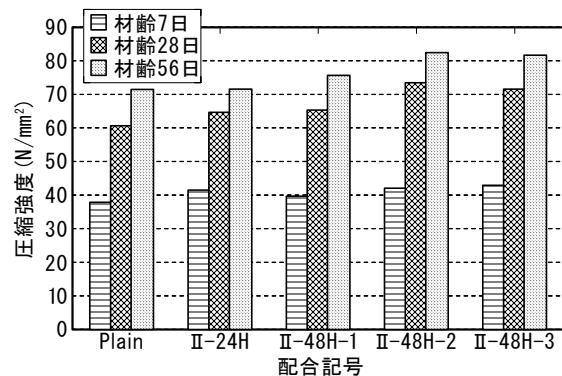
図-13 圧縮強度試験結果
