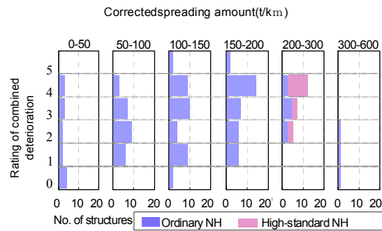
図-5 推定塩化物凍結防止剤散布量とスケーリング劣化グレード目視評価点（地覆車道側面）の比較[2]
