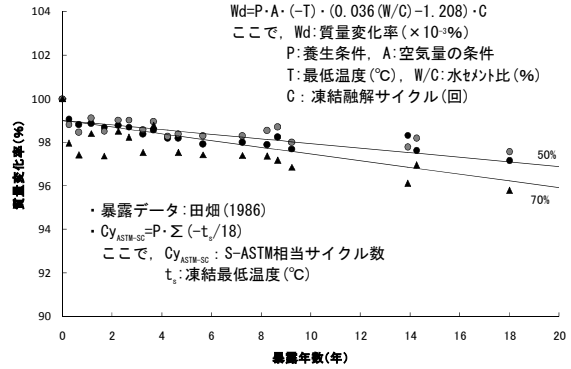
図-7 スケーリングの予測結果と屋外暴露試験との対応
