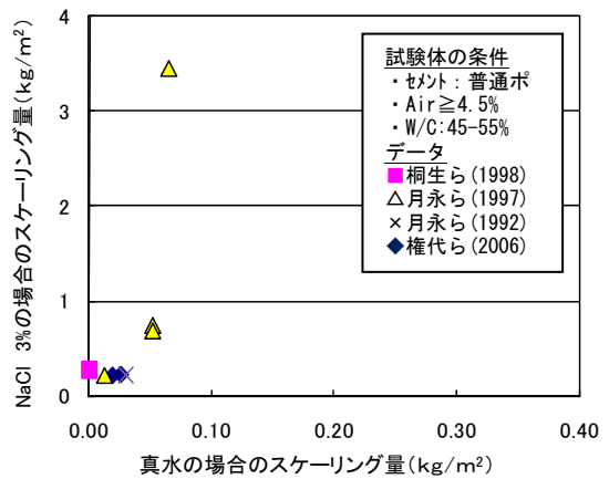
図-8 既往のスケーリング試験結果のまとめ (ASTM C672の場合)
