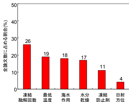
図-2 論文で採用されている主要な環境要因[1]
