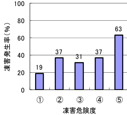
図-3 凍害危険度と道路橋の凍害発生率[3]
