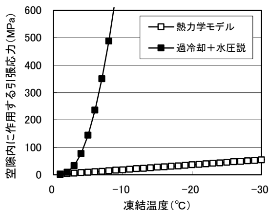
図-9 空隙内に作用する水分凍結による引張応力 (低飽水度)
