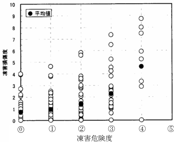
図-4 凍害危険度と凍害損傷度の関係[4]
