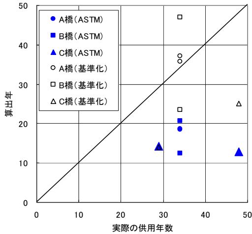
図-6 実構造物の実際の供用年数と予測手法により求めた算出年の関係[1]
