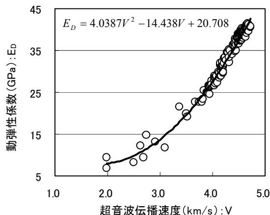
図-10 超音波伝播速度と動弾性係数の関係[5]
