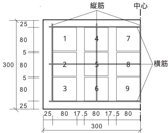
図 - 3 表面気泡と反発度の測定箇所(単位 : mm)
