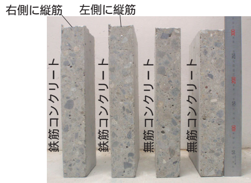
写真 - 4 鉄筋コンクリートと無筋コンクリートの断面の粗骨材の分布(120s)
