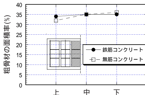
図 - 19 鉄筋コンクリートと無筋コンクリートの断面の粗骨材の面積率(右側に縦筋)(120s)
