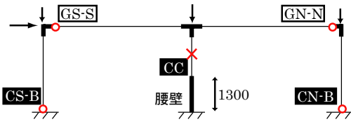
図-10 破壊モード混在型の建物モデル (Mモデル)
