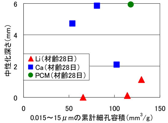
図-6 0.015~15 μm の累計細孔容積と中性化深さの関係 (促進 91 日)
