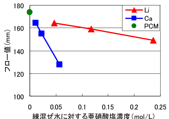
図-1 亜硝酸塩濃度とフロー値の関係
