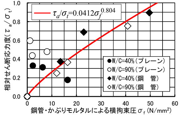
図-5 最大耐力時における支圧部側面のせん断抵抗成分と横拘束圧との関係
