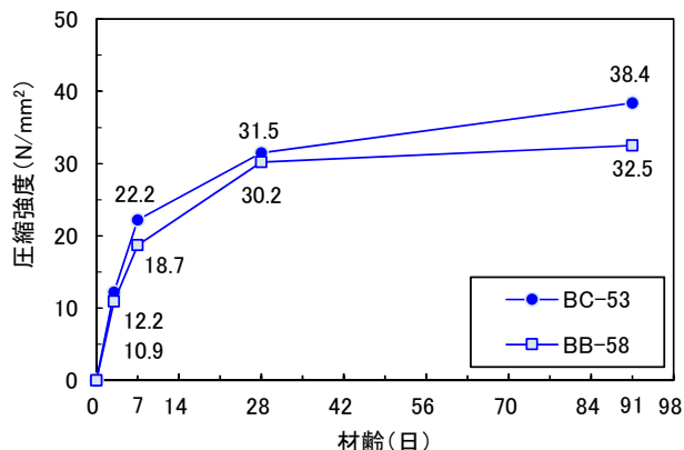
図-2 圧縮強度の比較
