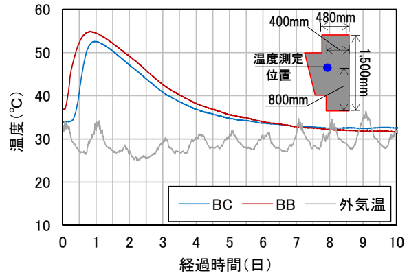
図-8 コンクリートの内部温度の比較
