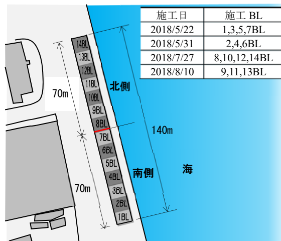
図-3 施工順序(平面図)およびコンクリートの打込み実績
